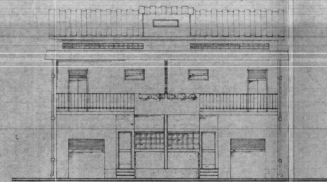
PROSPETTO POSTERIORE
