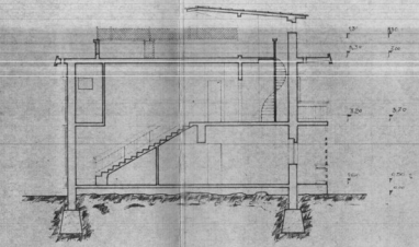
SEZIONE A-A
