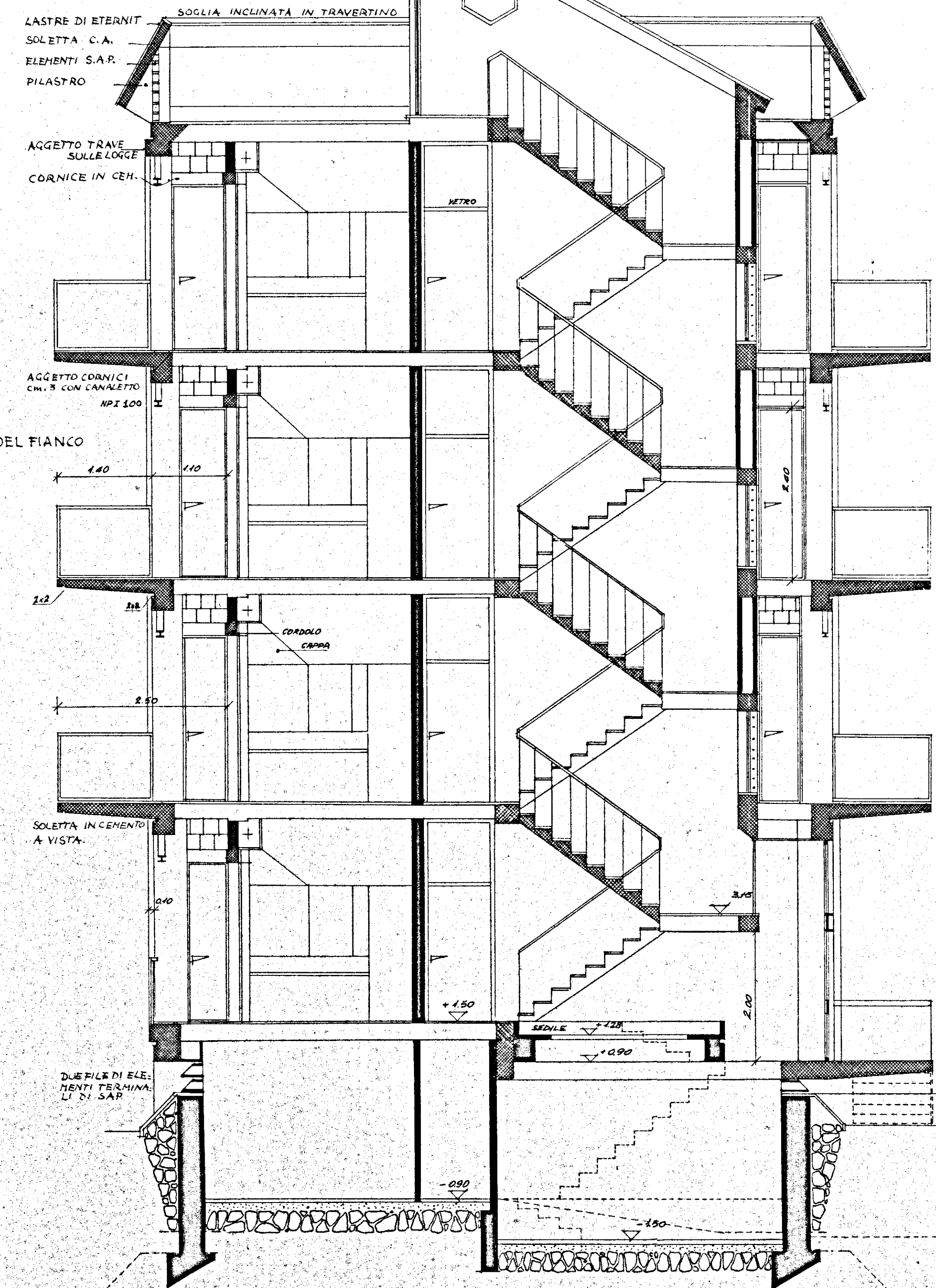
SEZIONE 1:50
