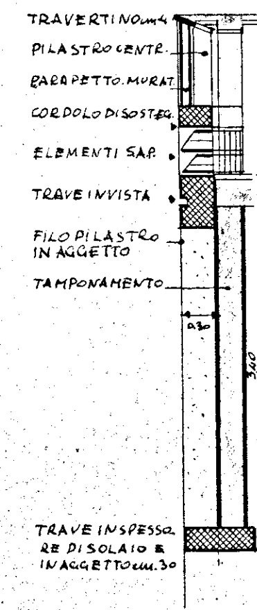
SEZIONE DEL FIANCO
