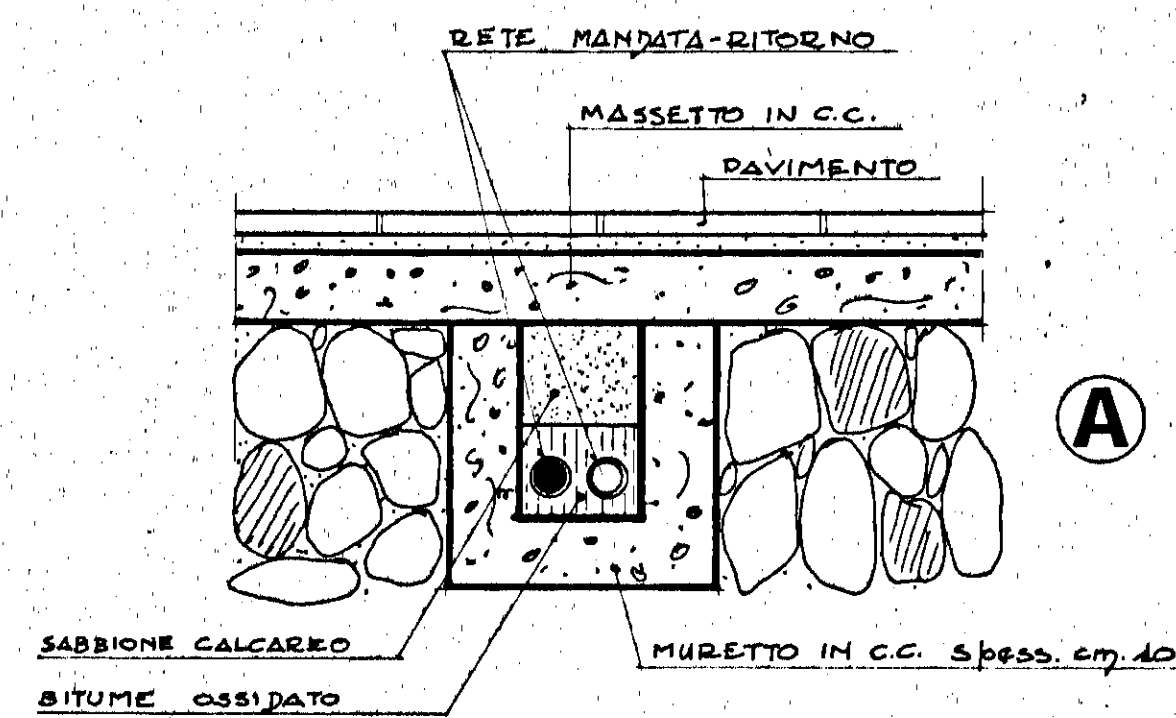
PARTICOLARE RETE INTERRATA IN CUNICOLO - Rapp. 1/10
