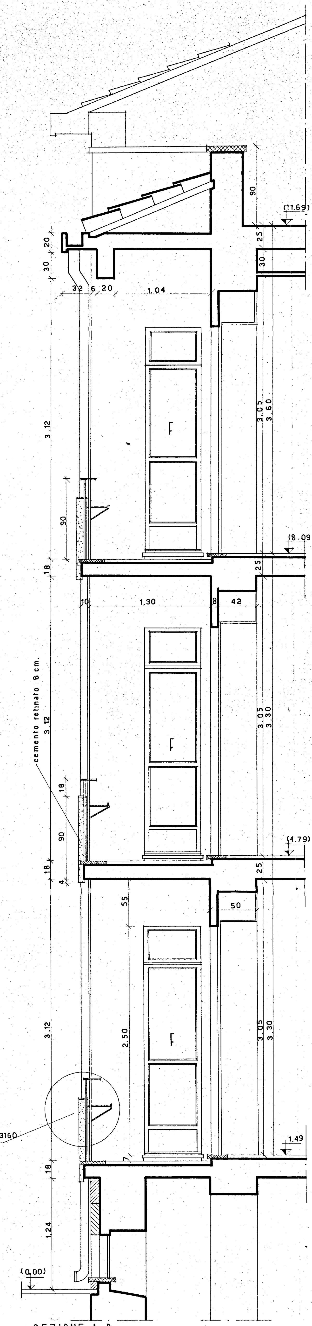
SEZIONE A-B
