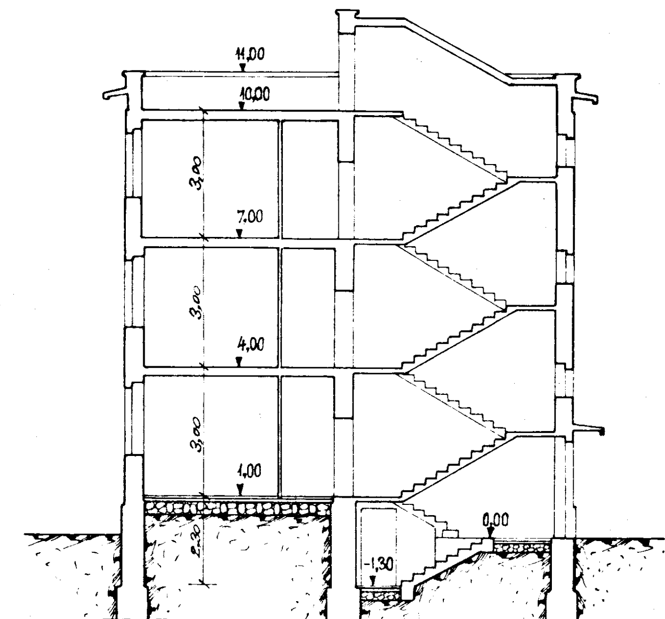
SEZIONE A-B
