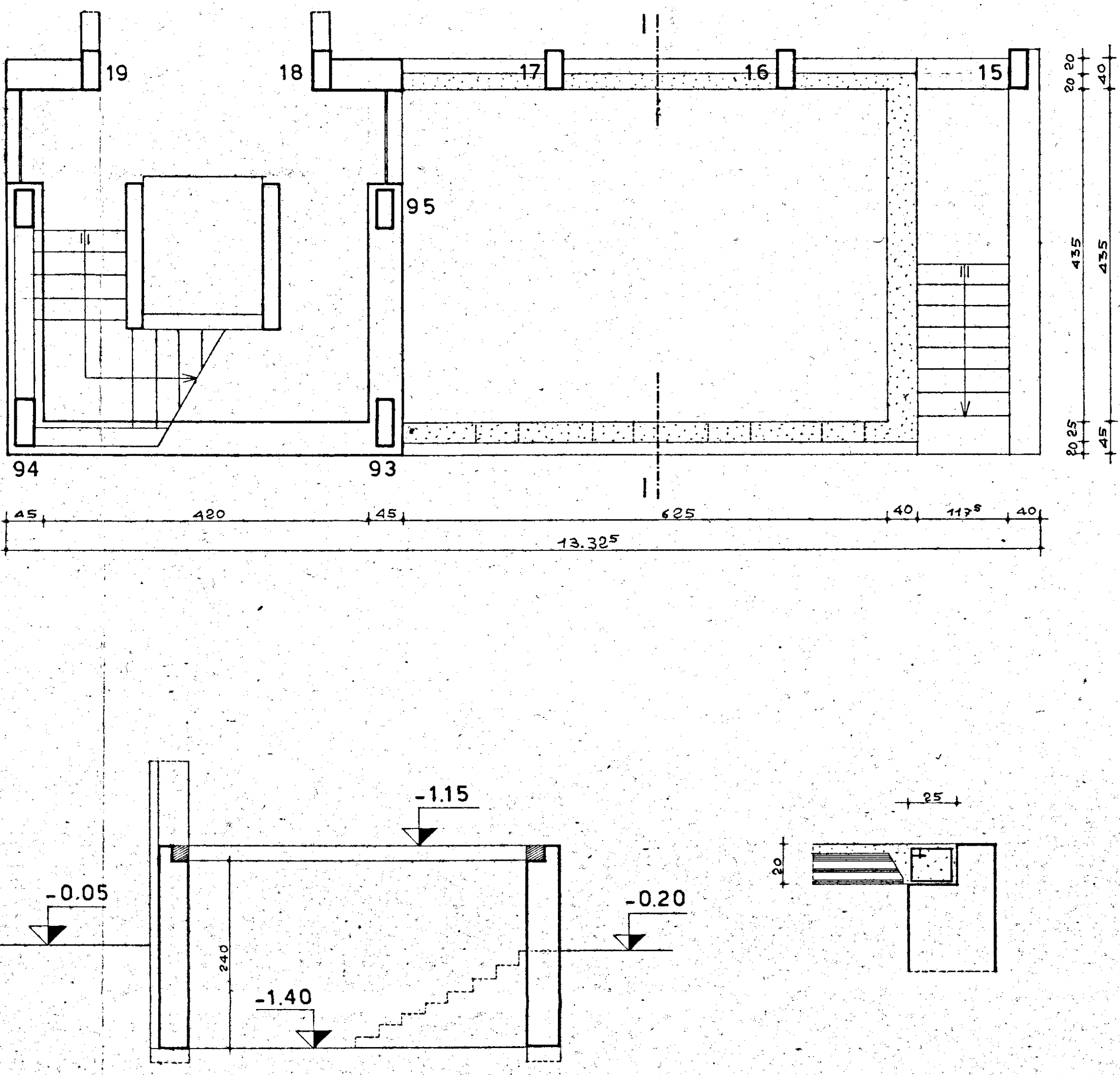
sez. 1 - 1
