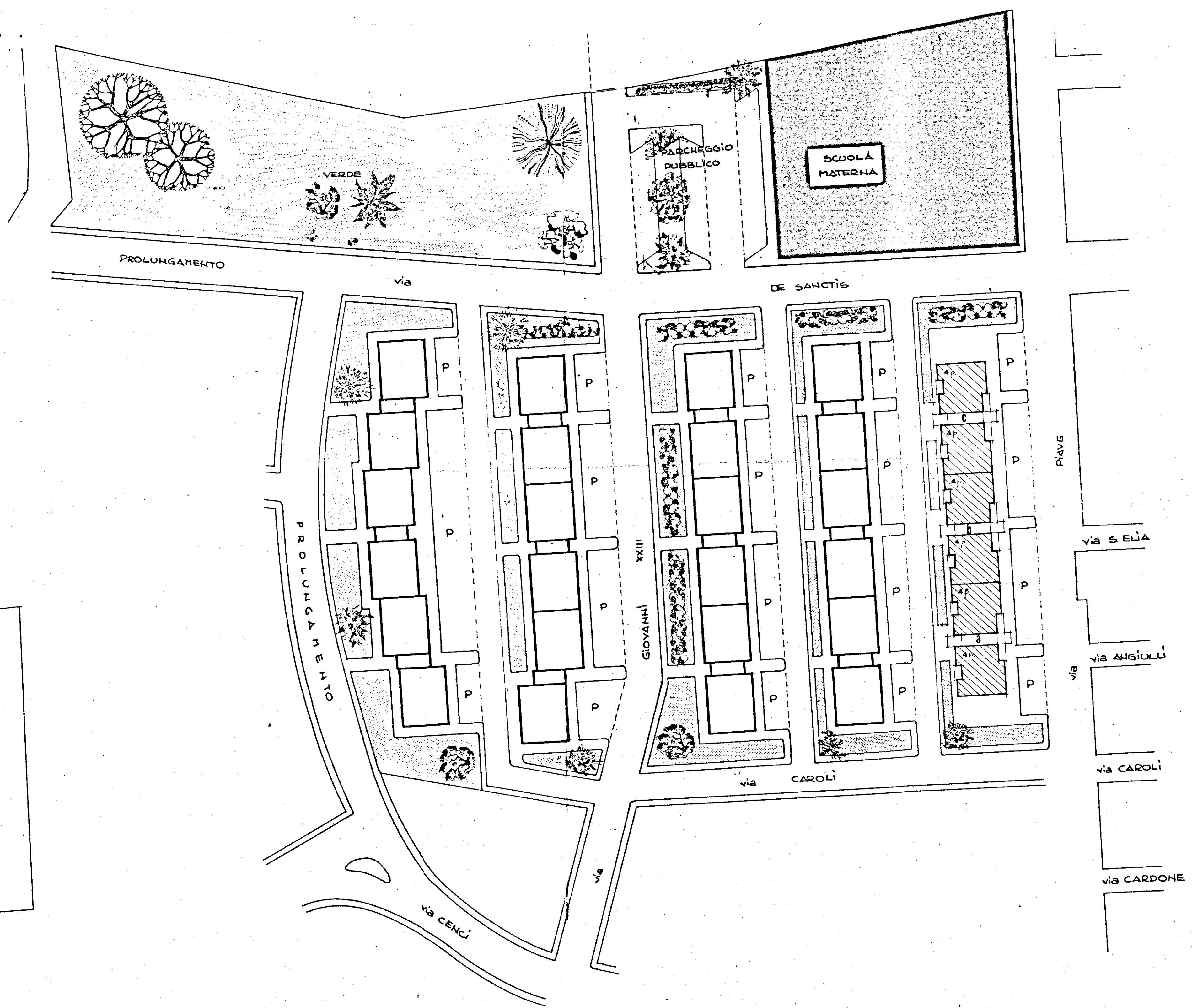
SCHEMA DI SISTEMAZIONE SPAZI ESTERNI E DEI FRONTI DEGLI EDIFICI SCALA 1:500
