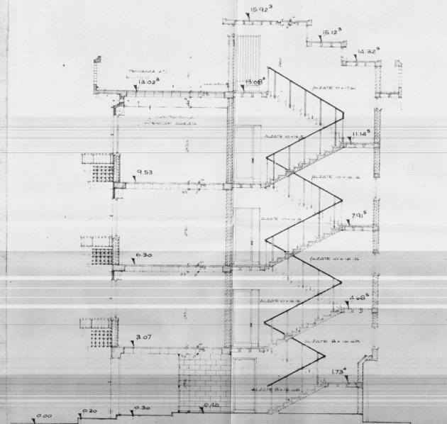
SEZIONE a-b
