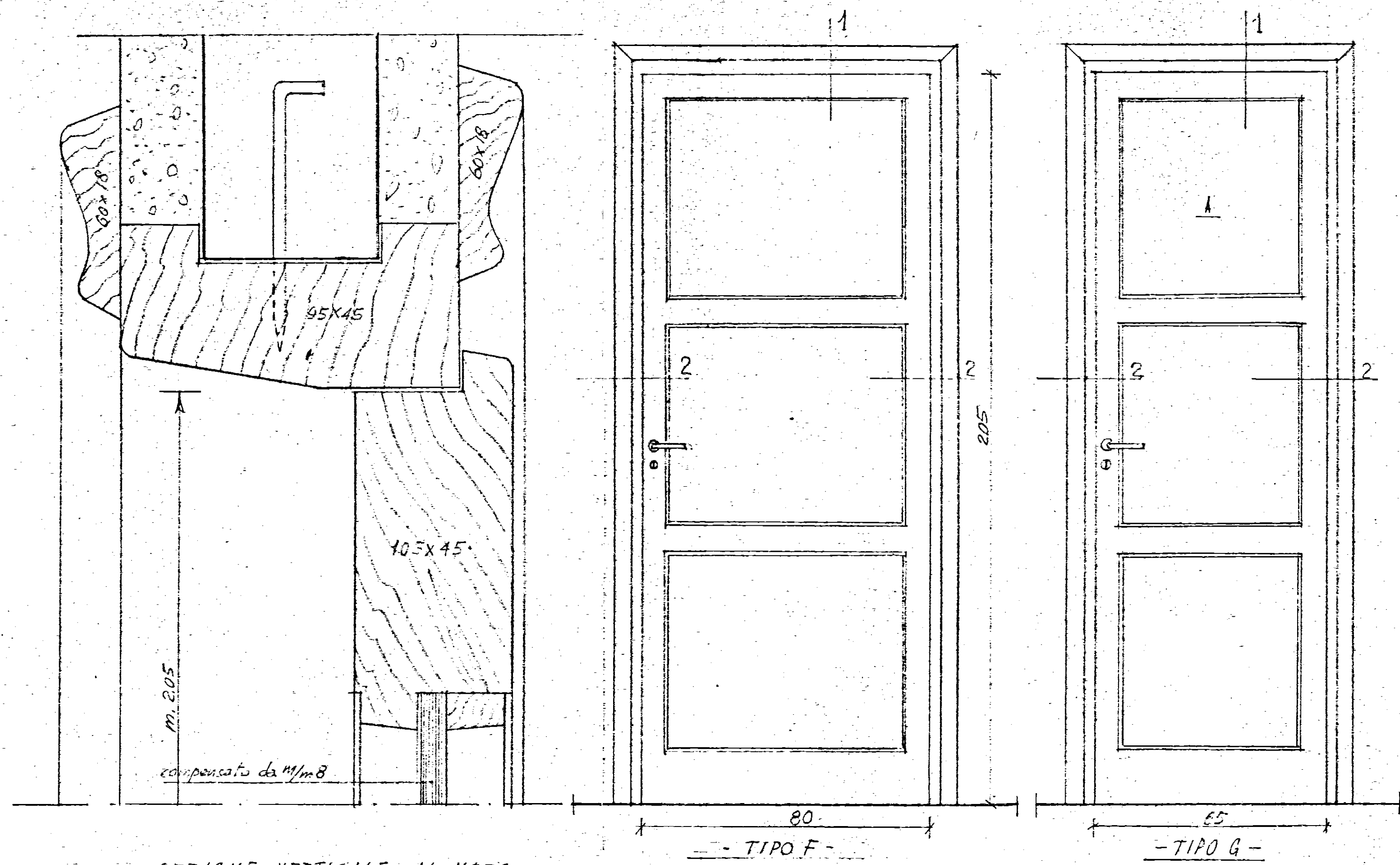
SEZIONE VERTICALE AL VERO.
