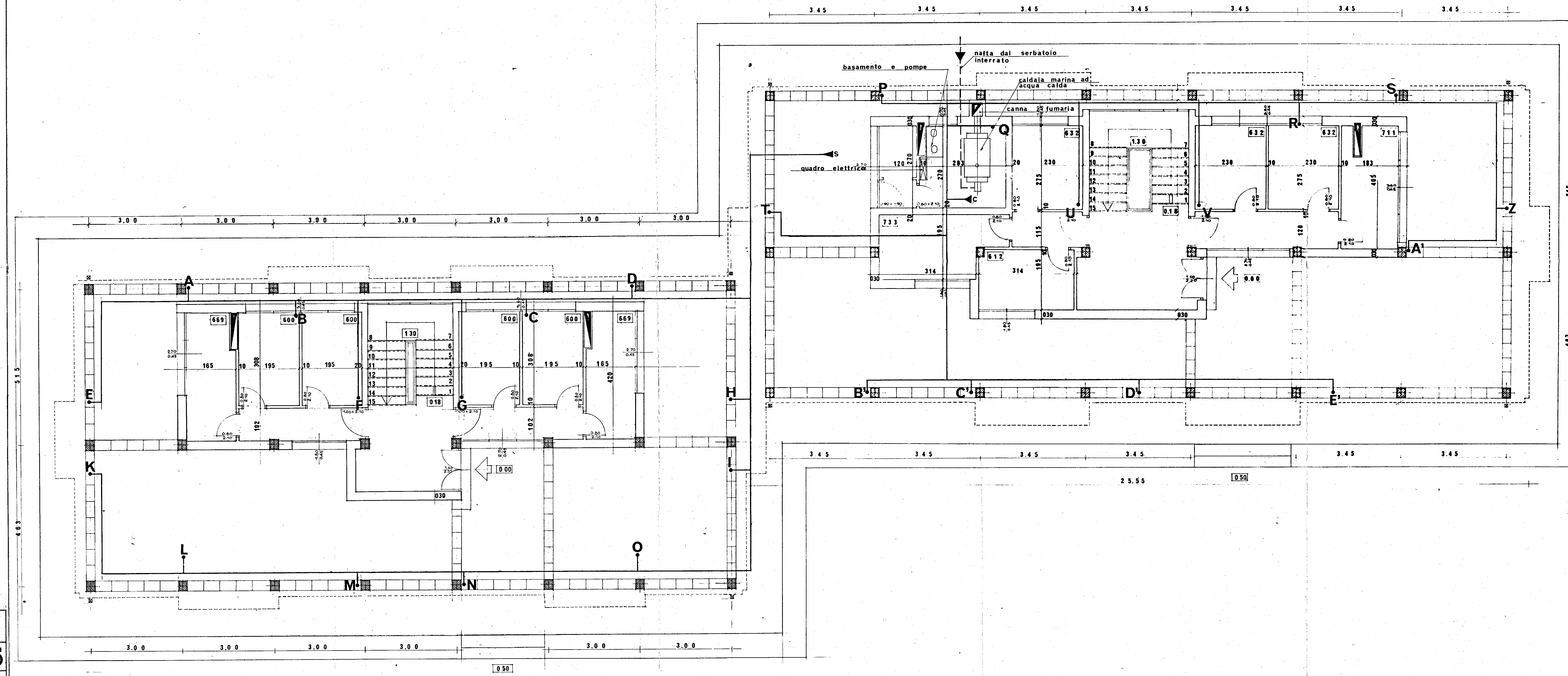
PIANTA DEL PIANO TERRENO rapp. 1:50
