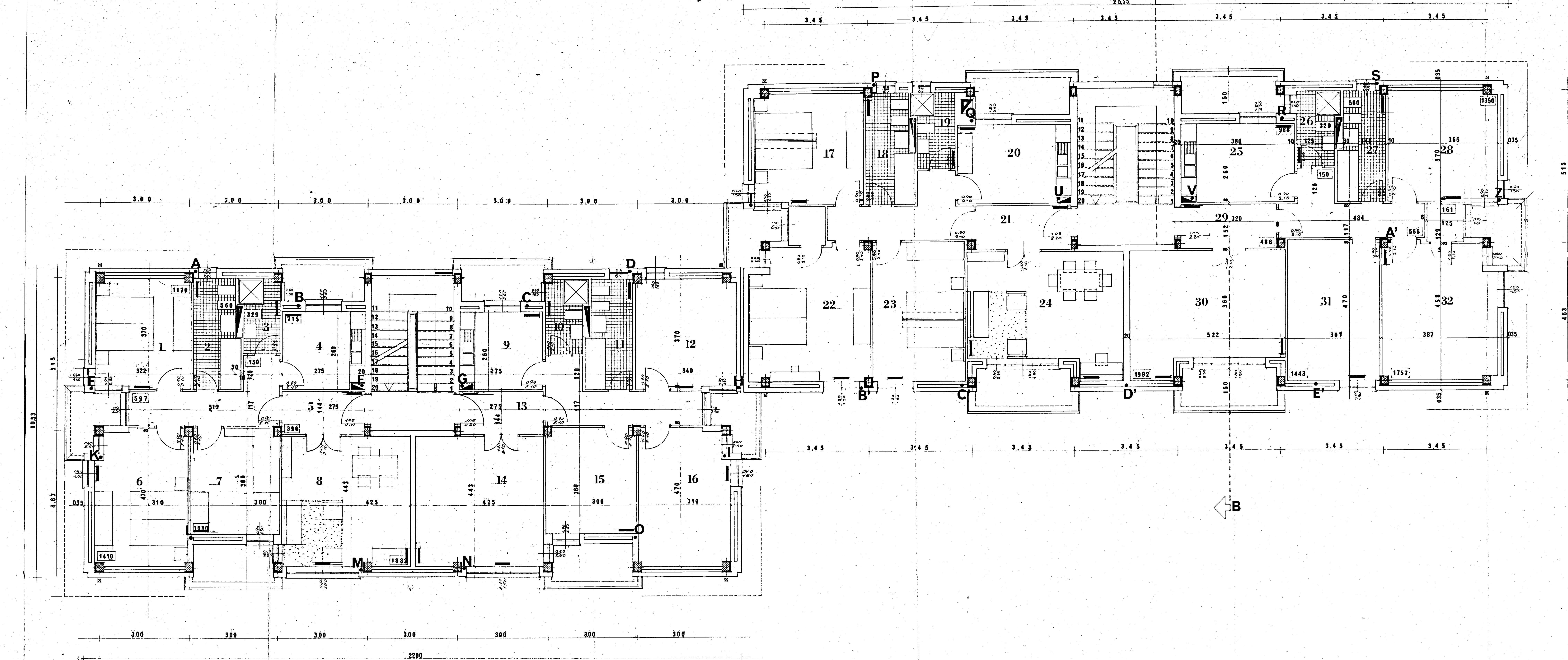
PIANTA DEL PIANO TIPO rapp. 1:50
