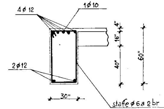
Sezione B-B
