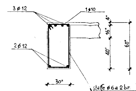
Sezione D-D
