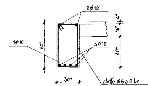
Sezione A-A
