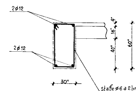
Sezione E-E
