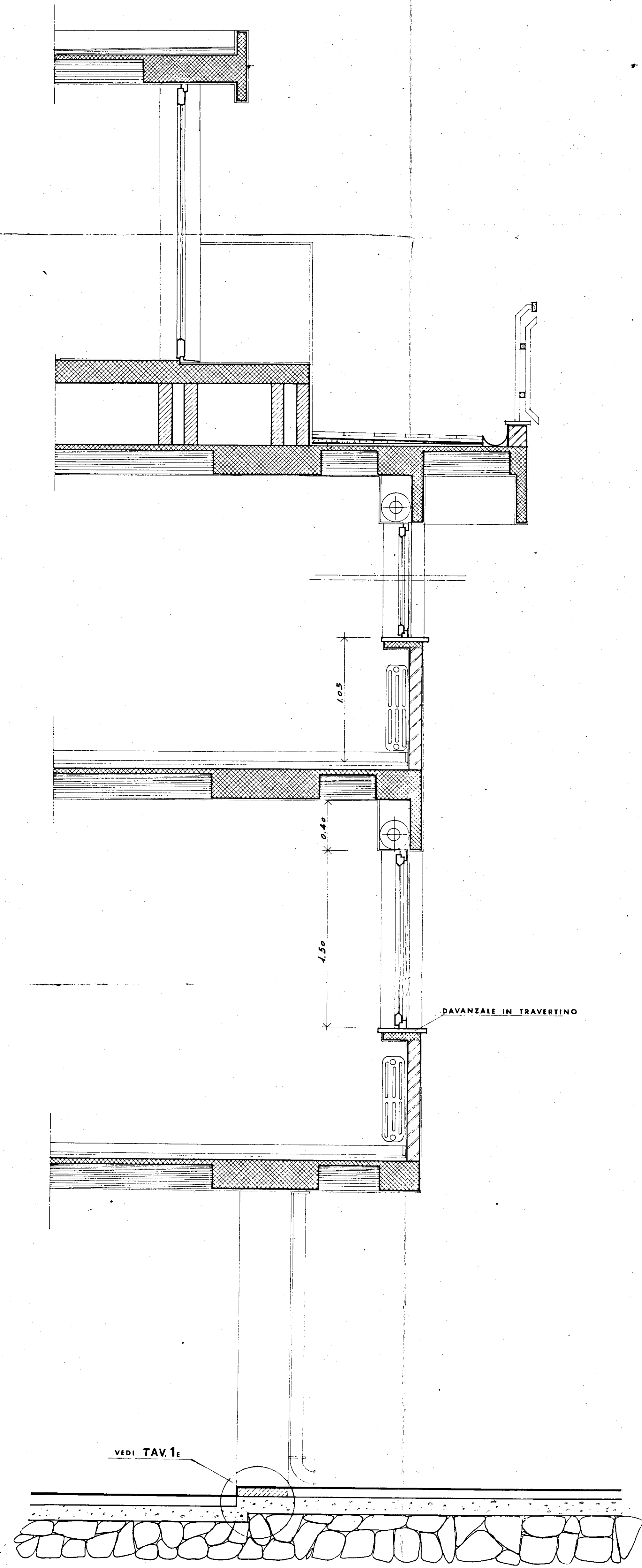
SEZIONI TIPO
