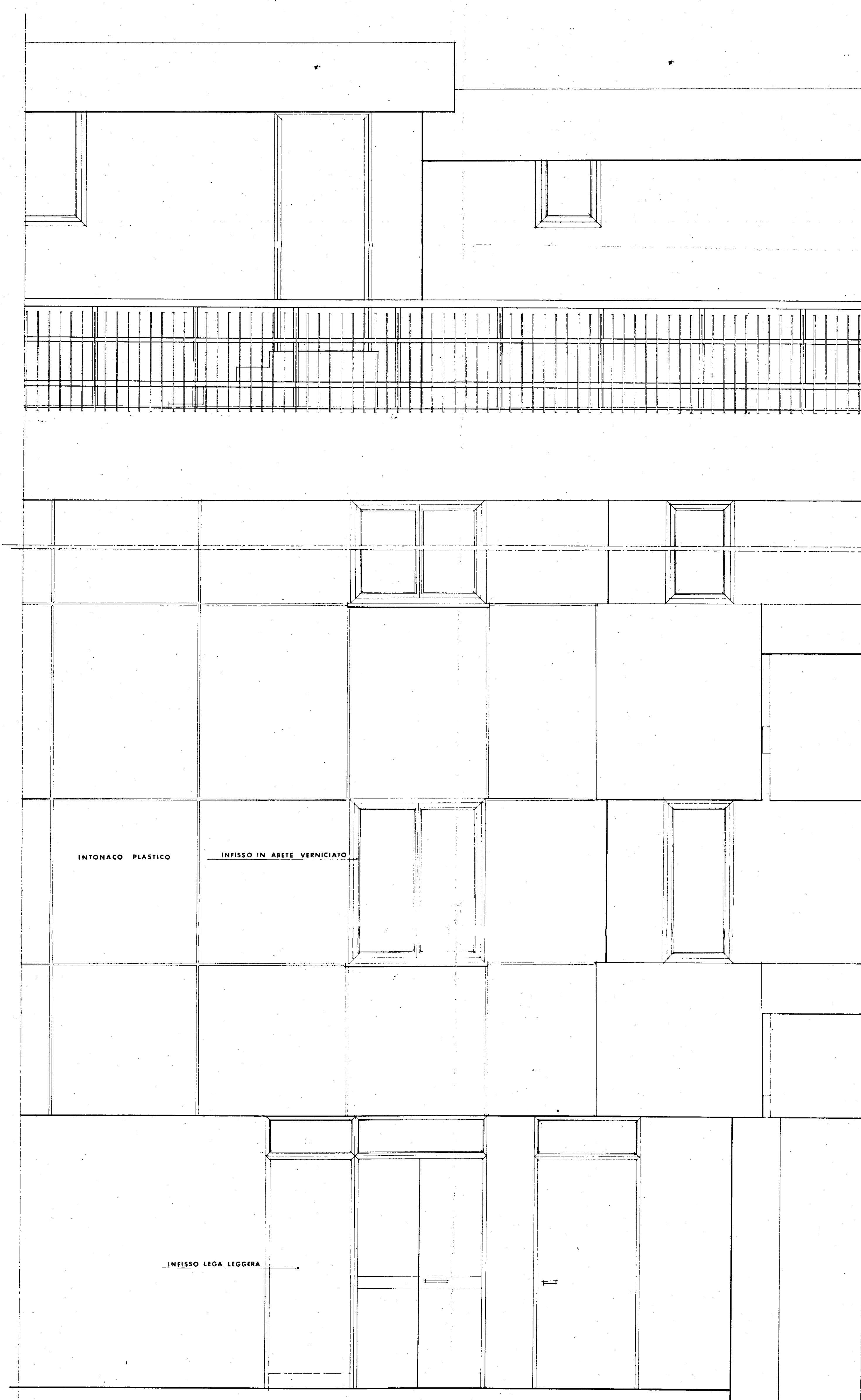
PROSPETTO
