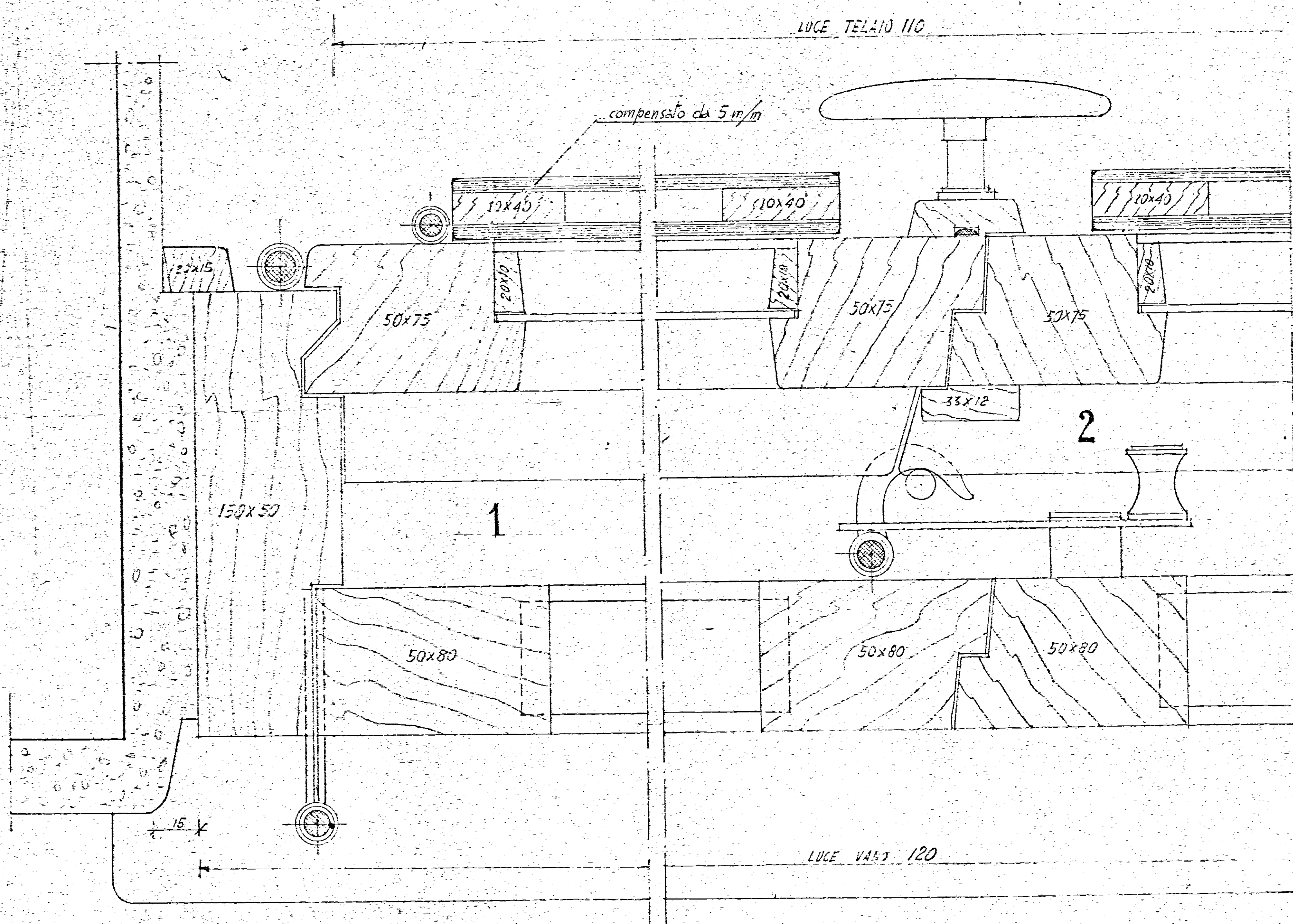
TIPO A LUCE VANO 120 LUCE TELAI 110 TIPO A* (lindierino) LUCE VANO 120 X 250 LUCE TELAI 110 X 245
