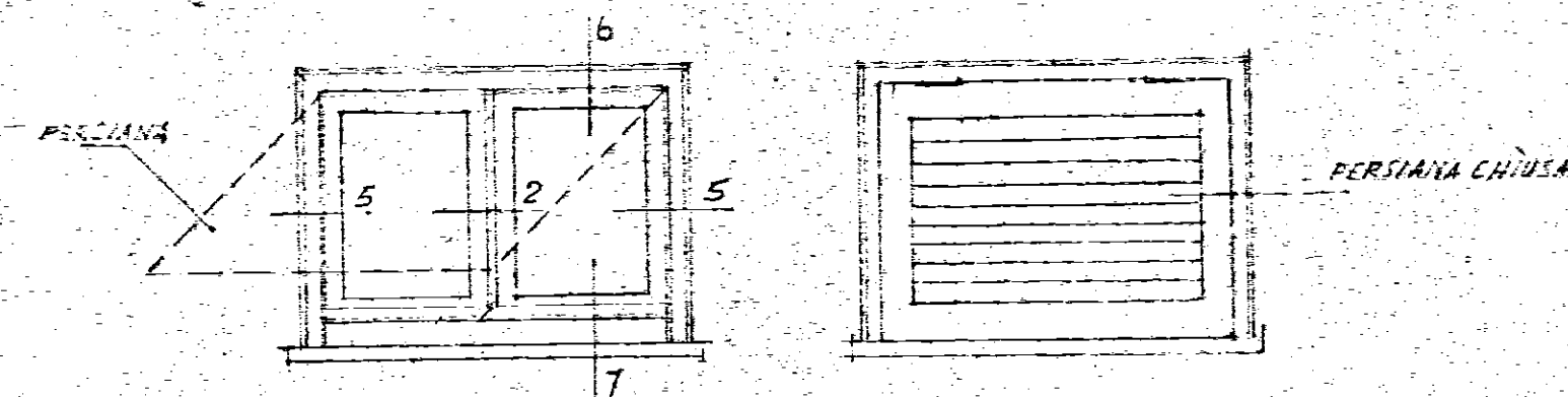
TIPO B LUCE VANO 100 X 70 LUCE TELAIO 90 X 58 5 TIPO B* LUCE VANO 115 X 70 LUCE TELAIO 105 X 58 5
