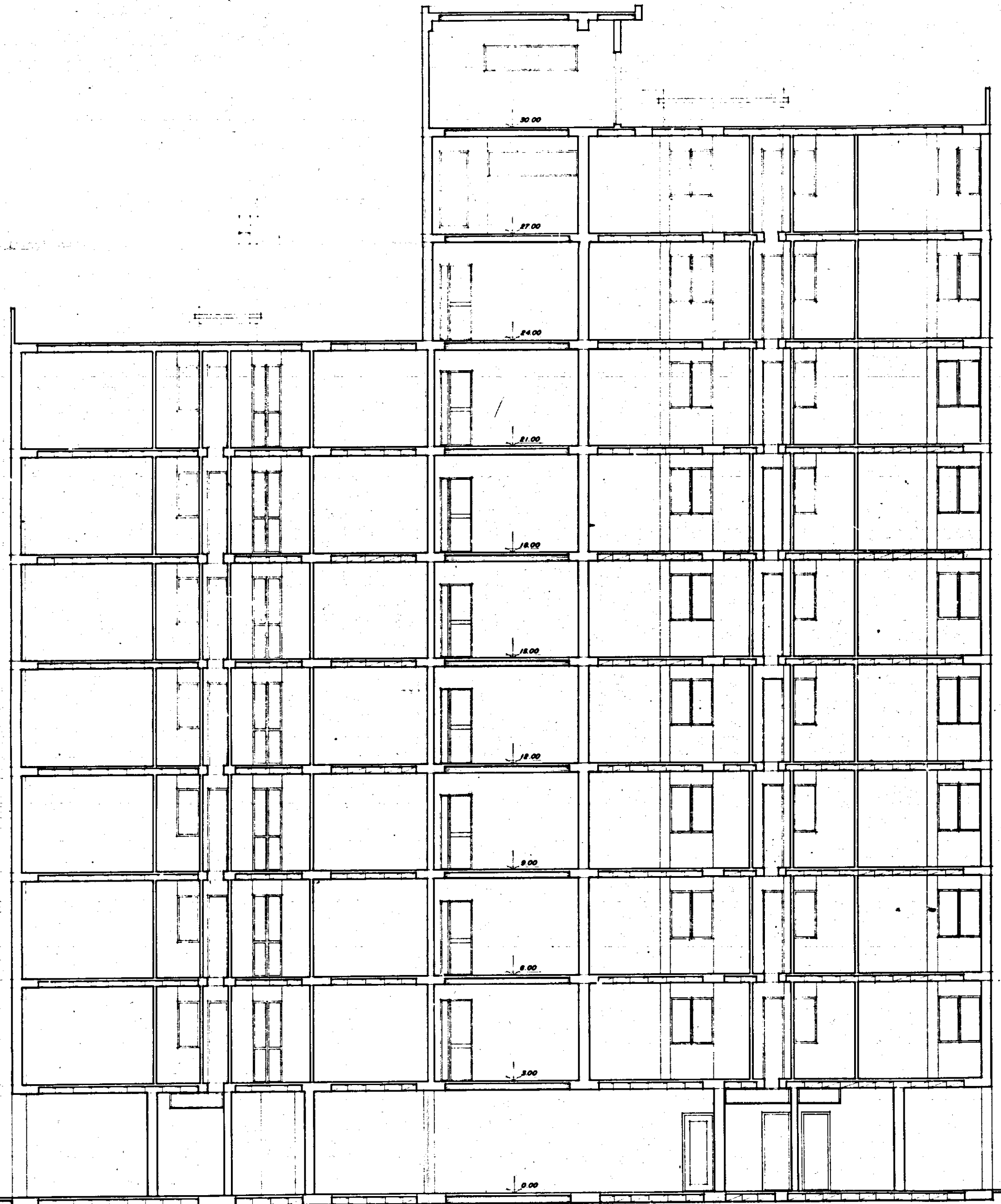
SEZIONE Y - Y
