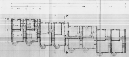
PIANTA PIANO TIPO
