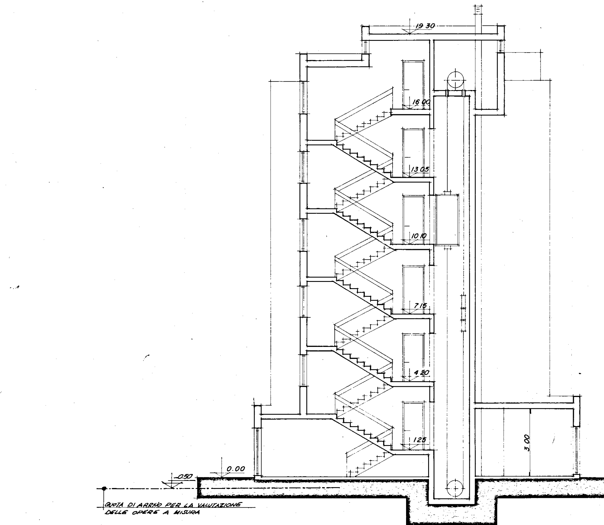
SEZIONE Y - Y
