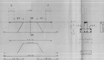
SEZIONE M - M
