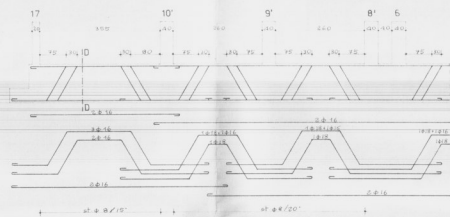
SEZIONE D - D
