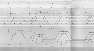
SEZIONE G - G
