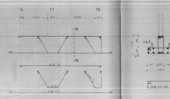
SEZIONE N - N
