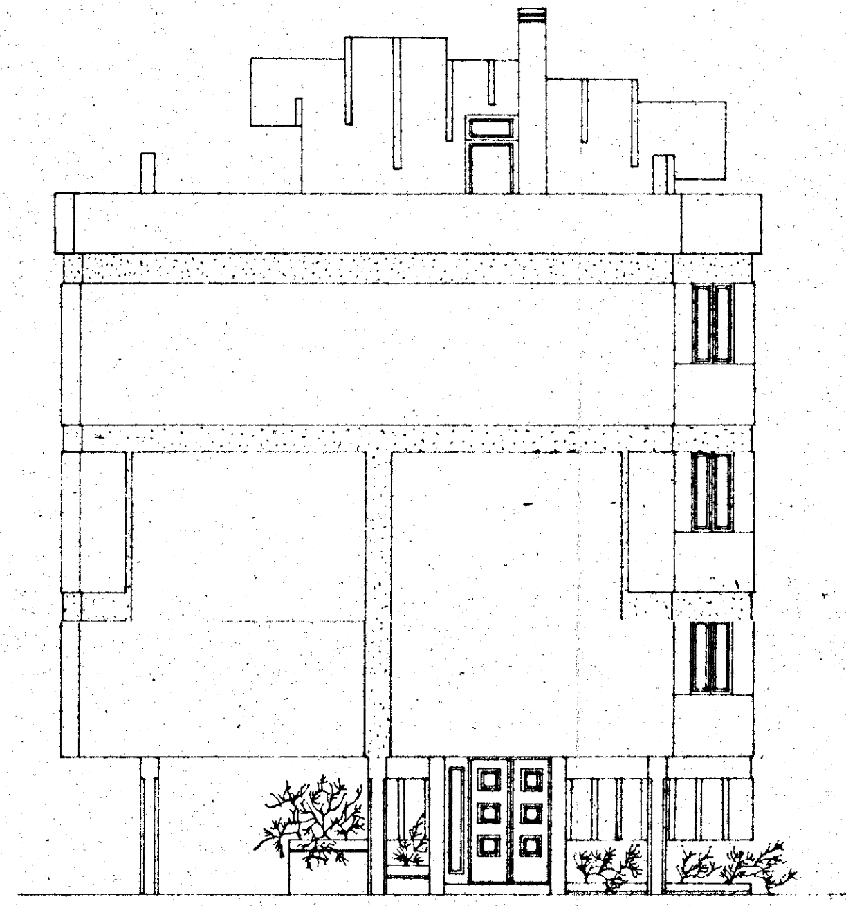
PROSPETTO LATERALE
