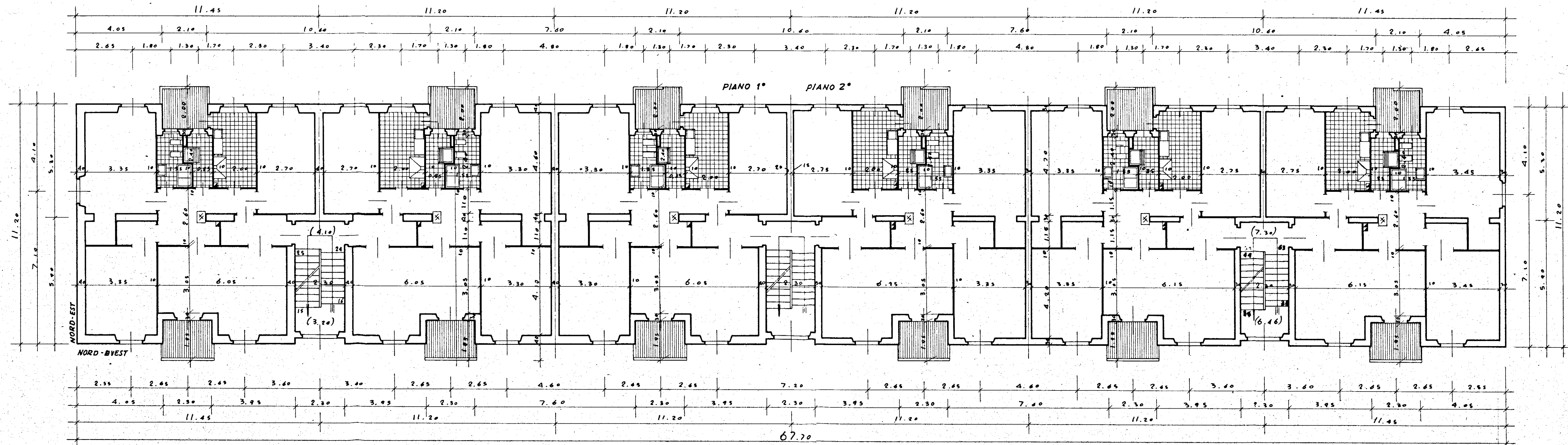
DIS. 161 PIANTE PIANO 1° E 2° RAPP. 1:100
