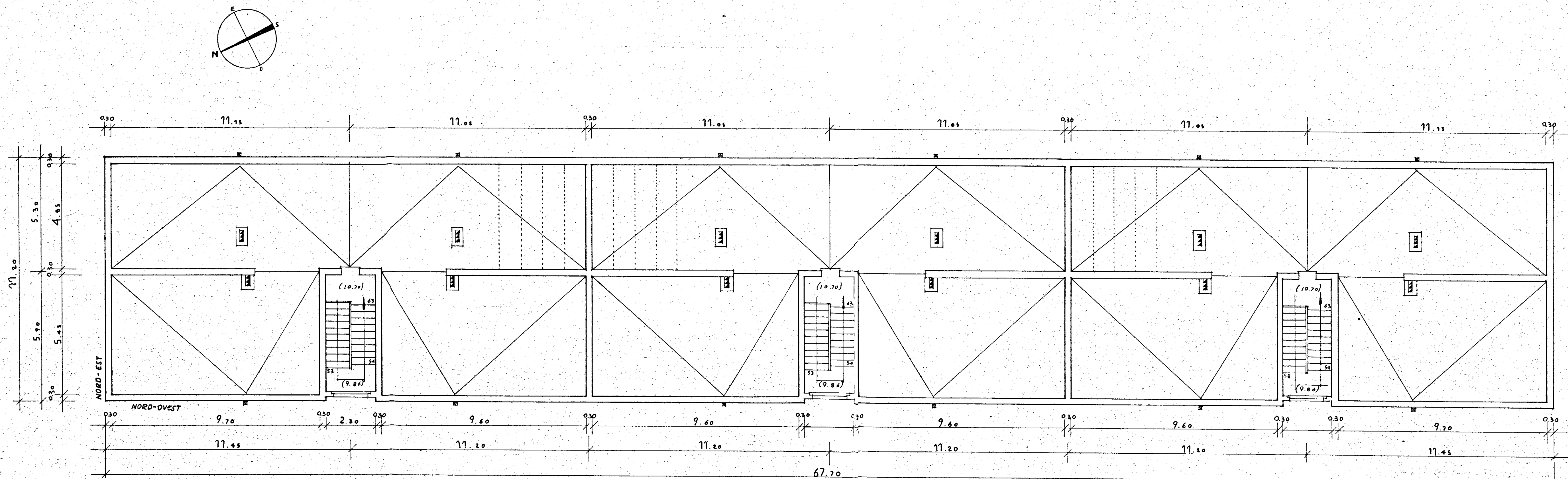
DIS. 162 PIANTA PIANO COPERTURA RAPP. 1:100
