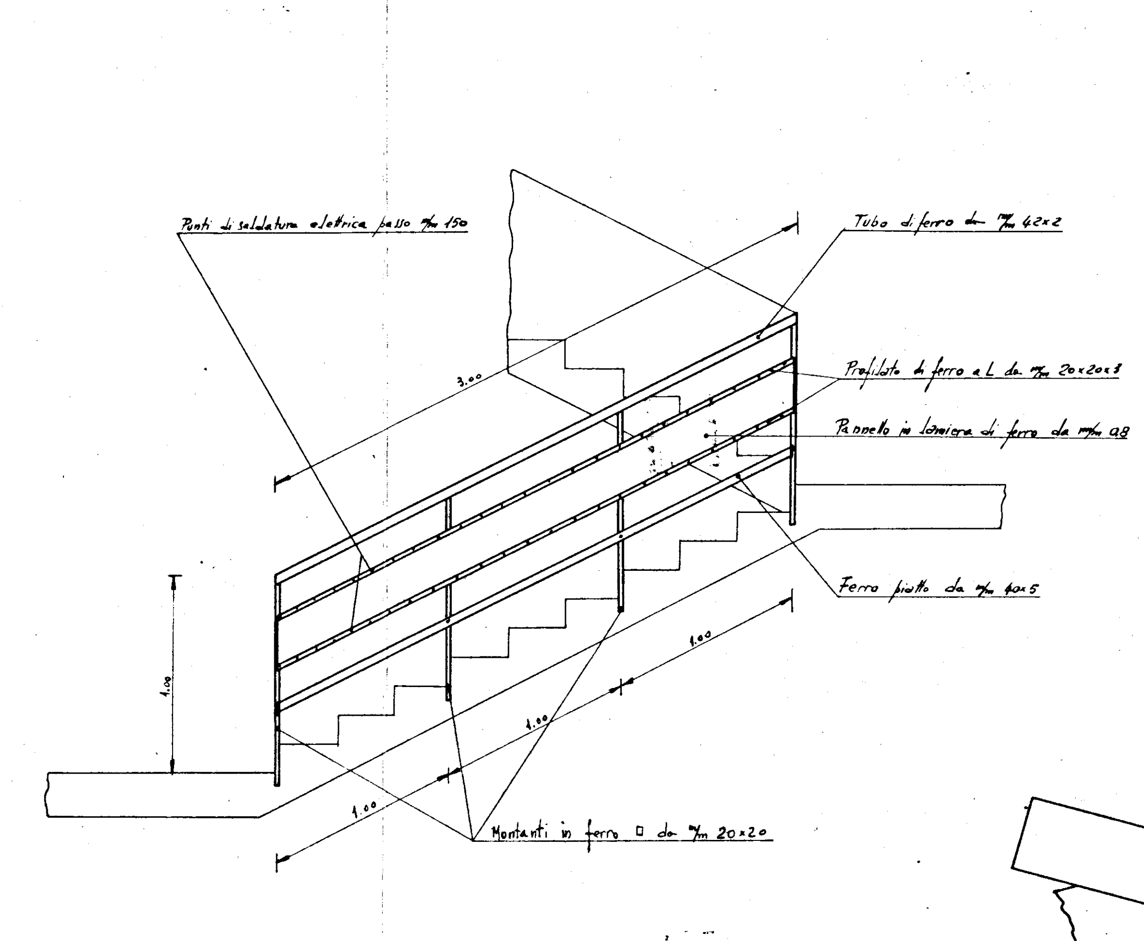
RINGHIERA PER SCALE SCALA 1:20
