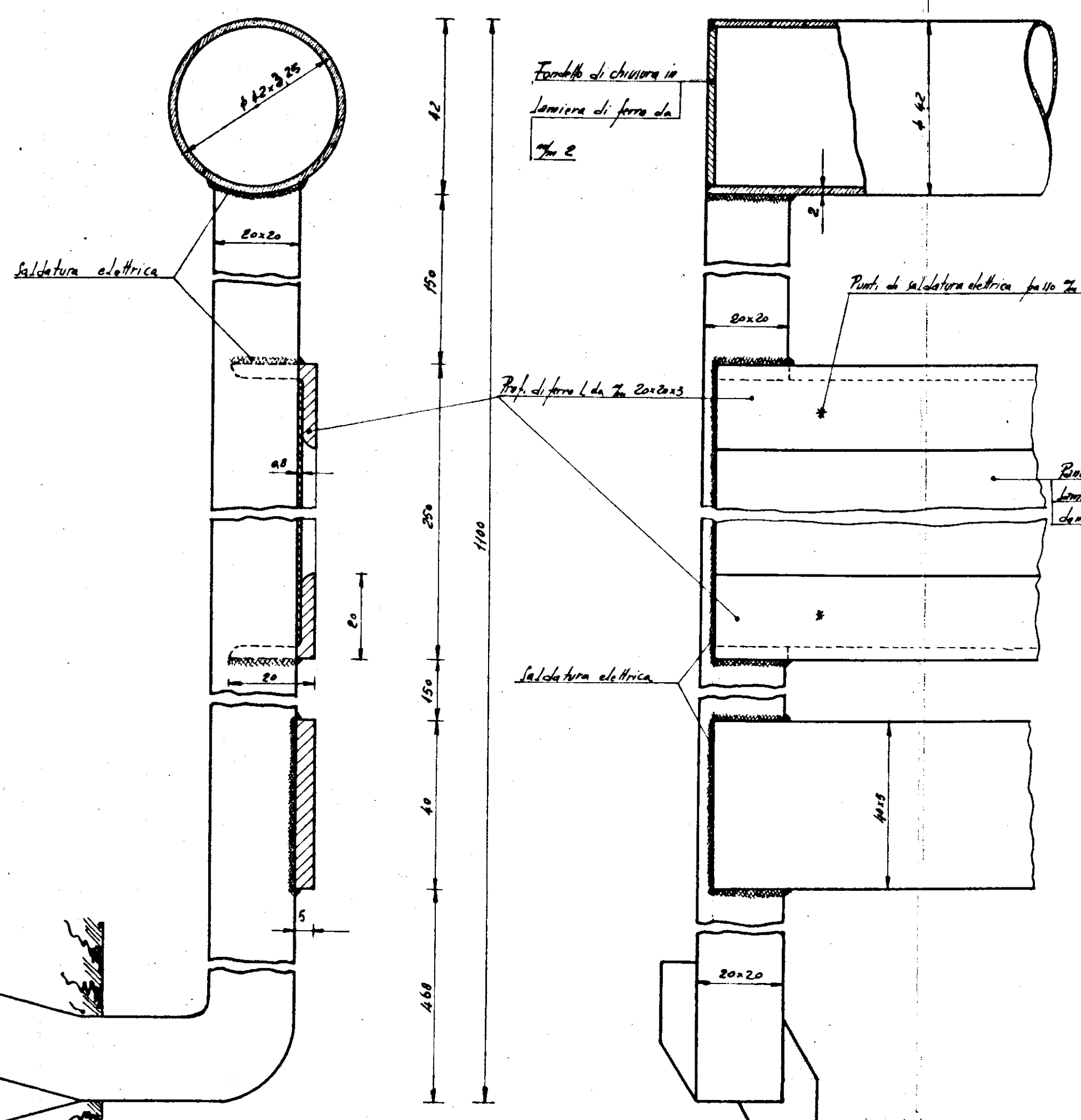
PARTICOLARE MONTANTE - SCALA 1:1
