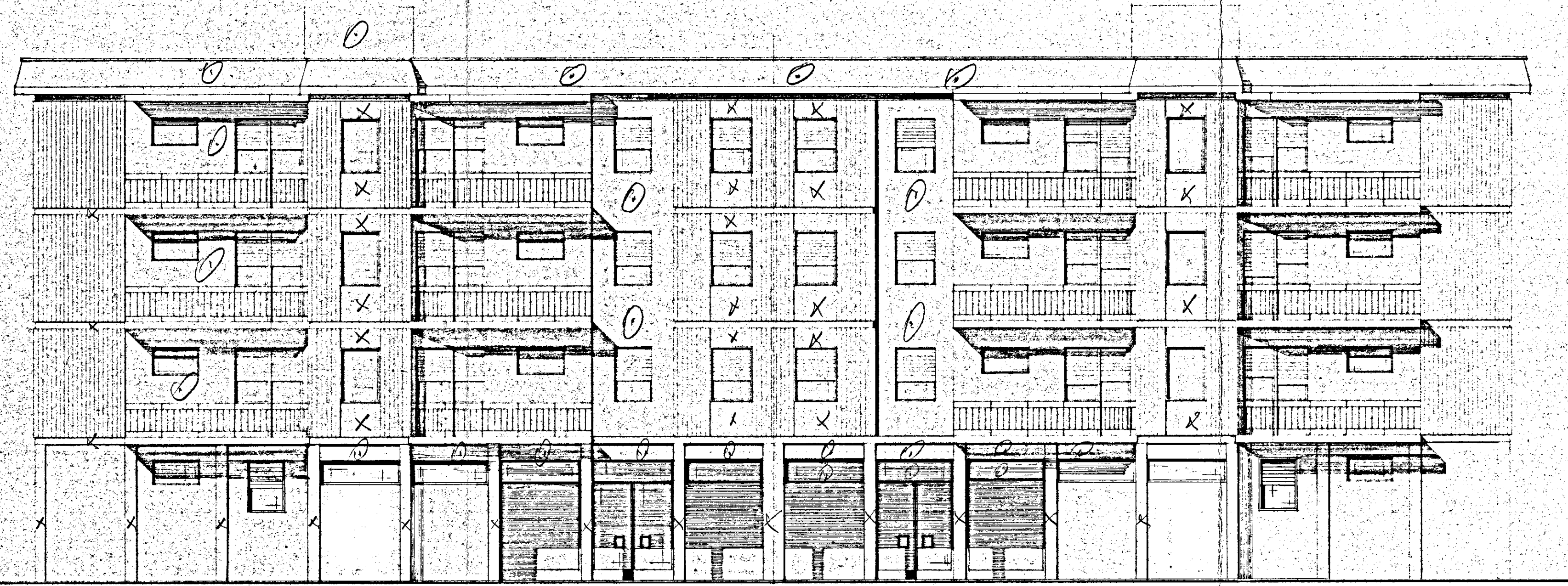
PROSPETTO 'A'
