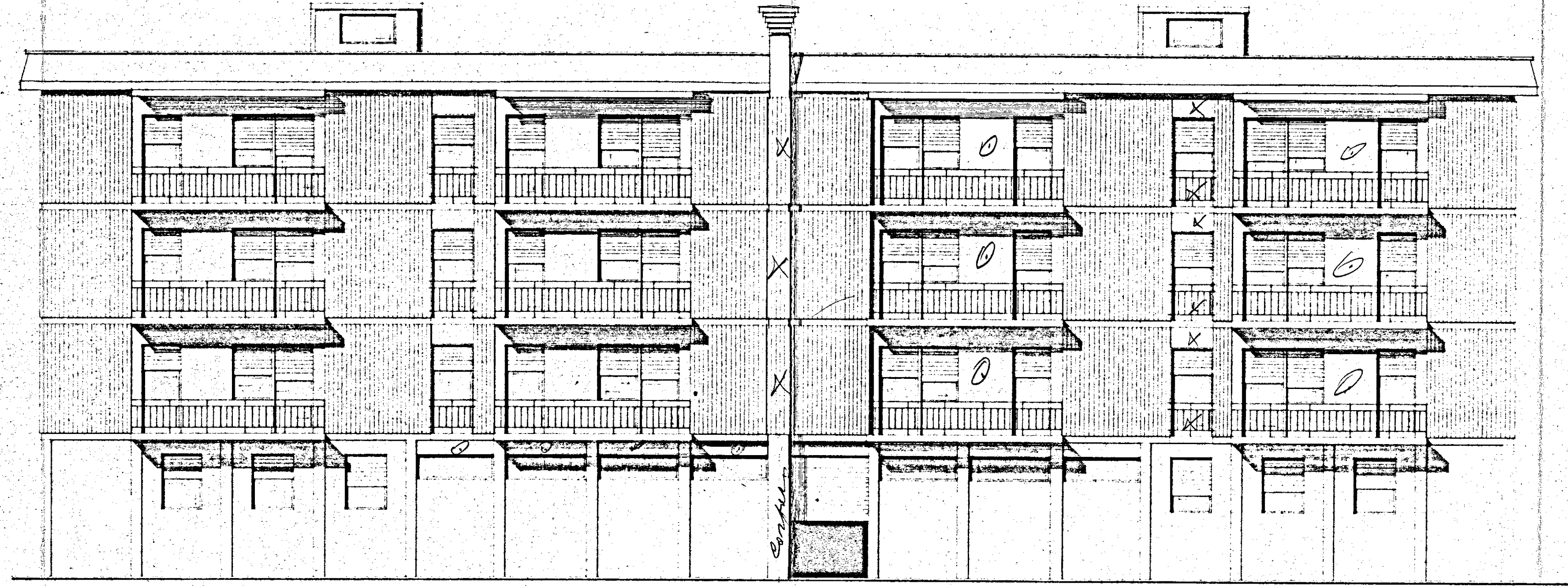
PROSPETTO 'C'
