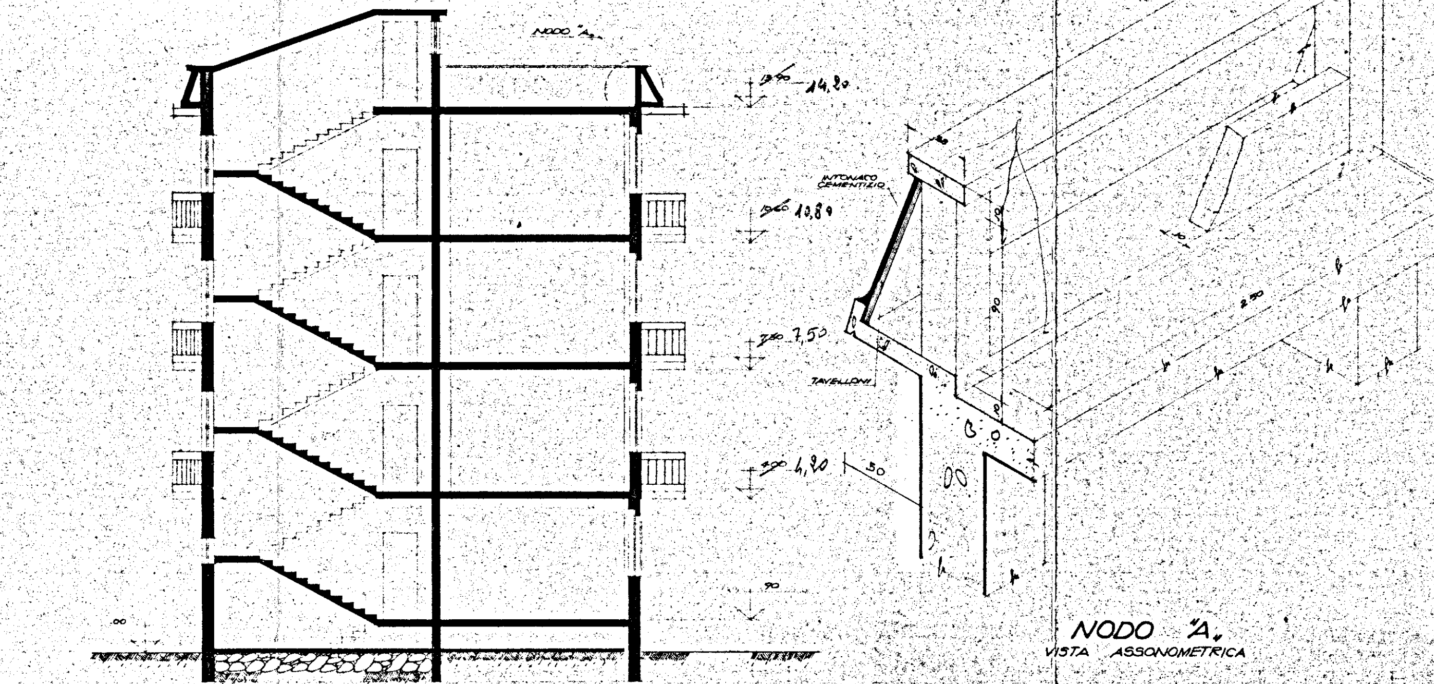
SEZIONE X-X
