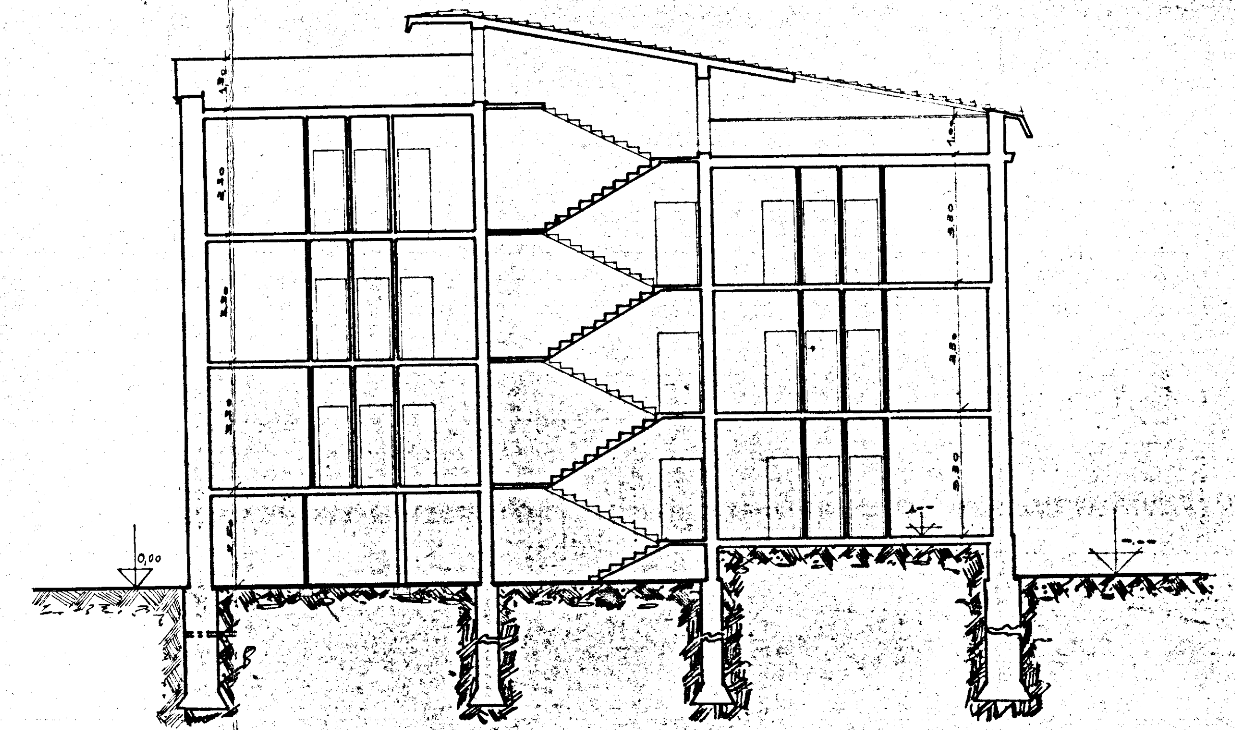
SEZIONE LONGITUDINALE
