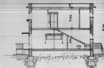
SEZIONE E-E'
