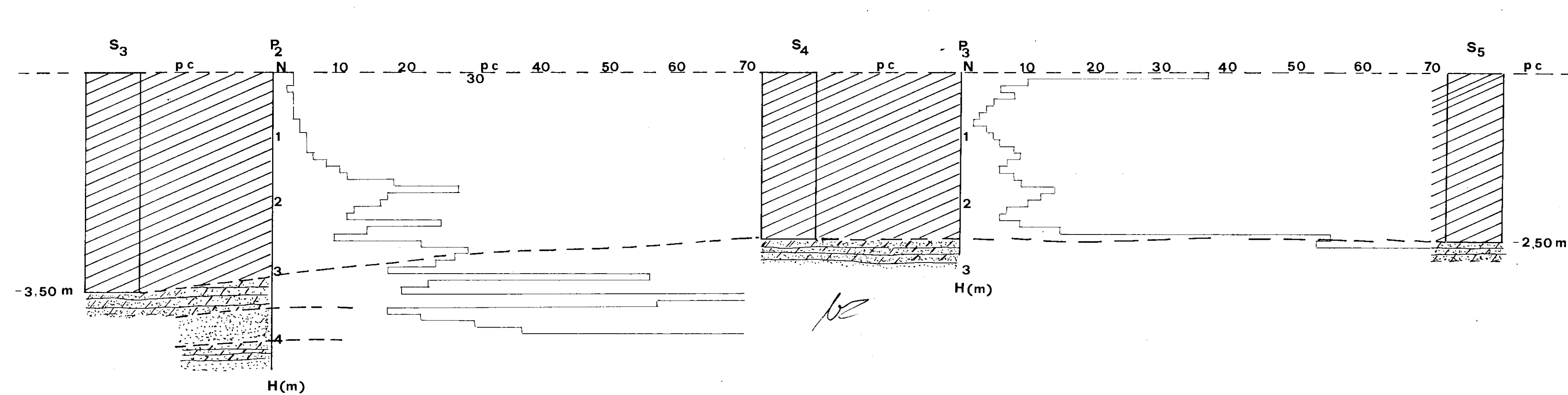
SEZIONE STRATIGRAFICA 2
