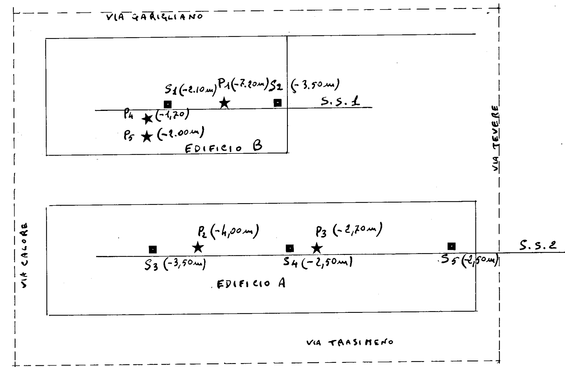
SCHEMA PLANIMETRICO scala 1:500
