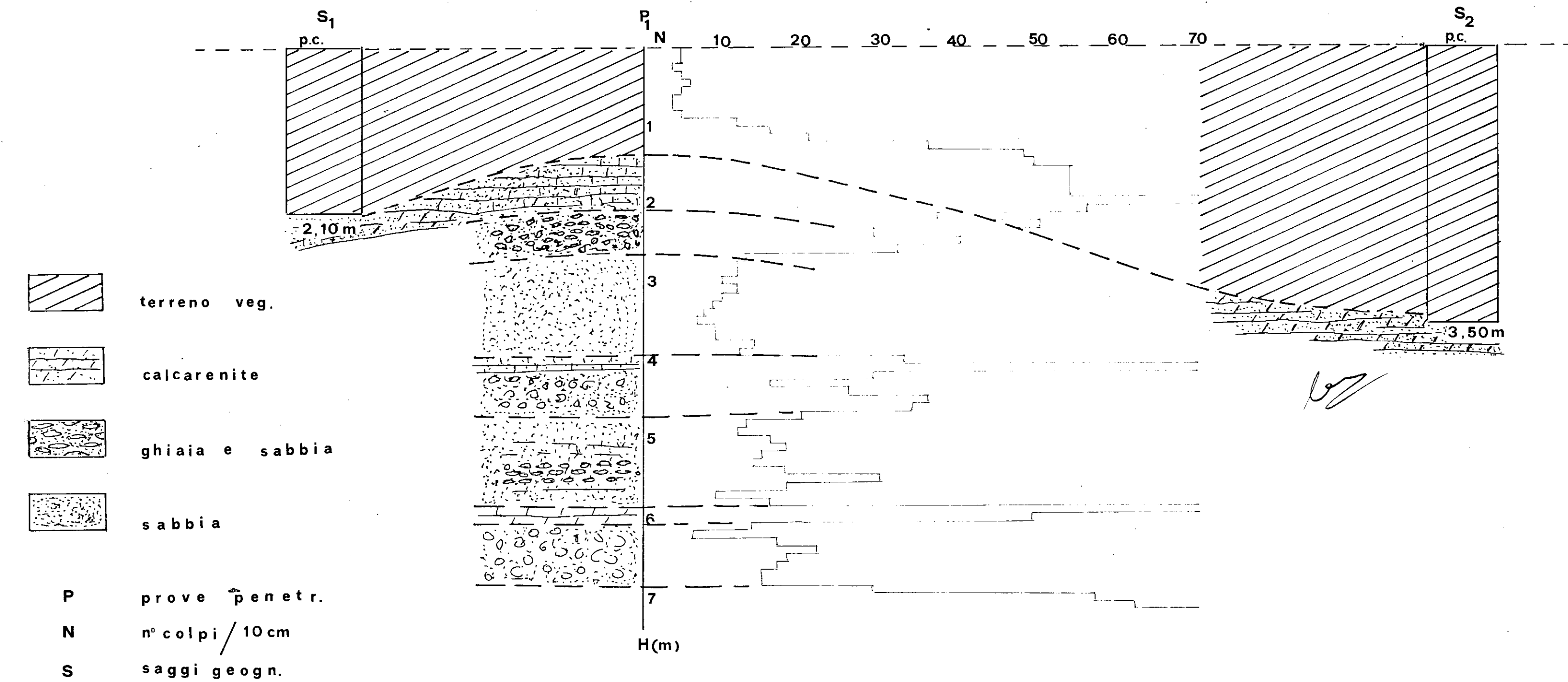
SEZIONE STRATIGRAFICA 1
