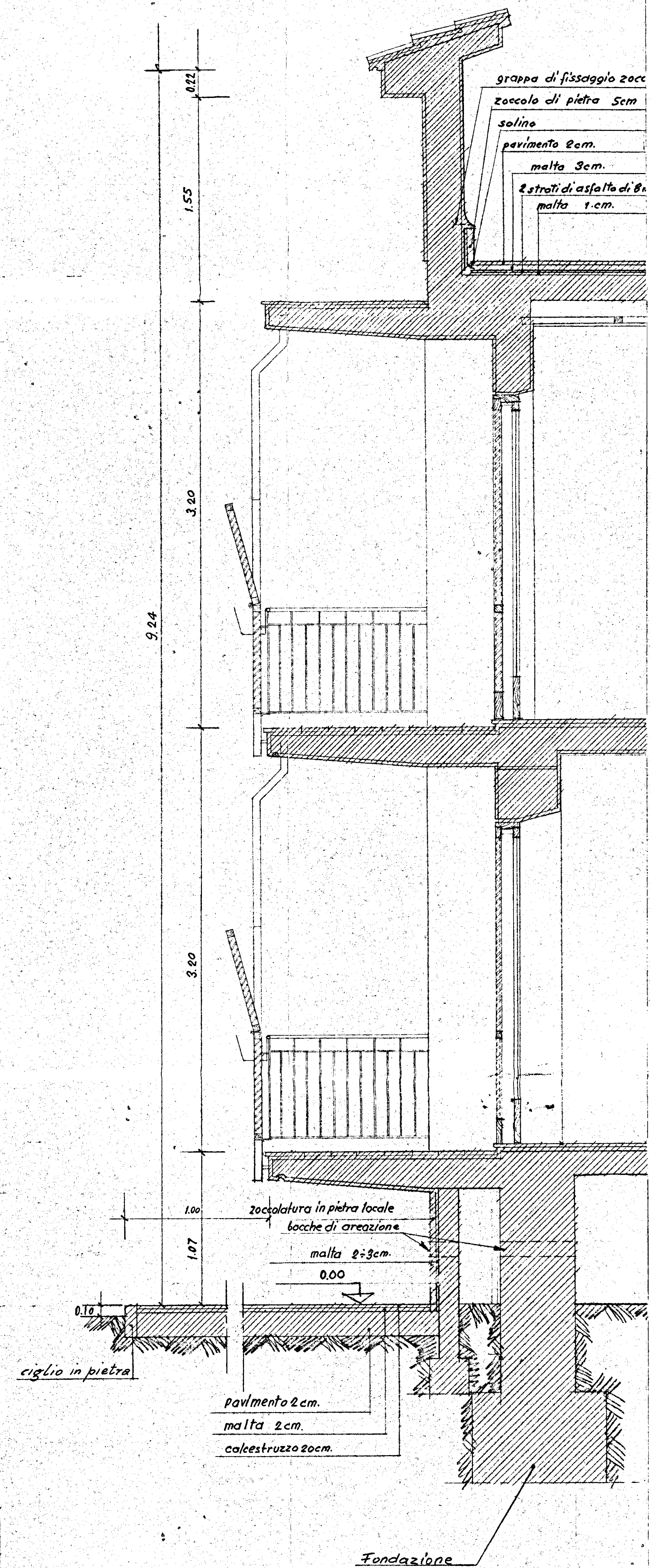
SEZIONE A-A
