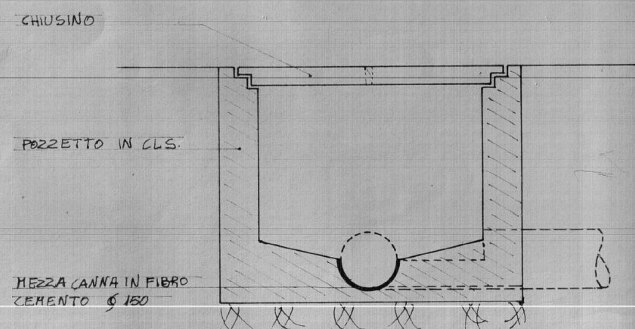
SEZIONE POZZETTO
