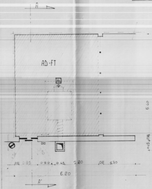
RILIEVO PIANTA CENTRALE TERMICA
