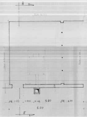
RILIEVO PIANTA CENTRALE TERMICA
