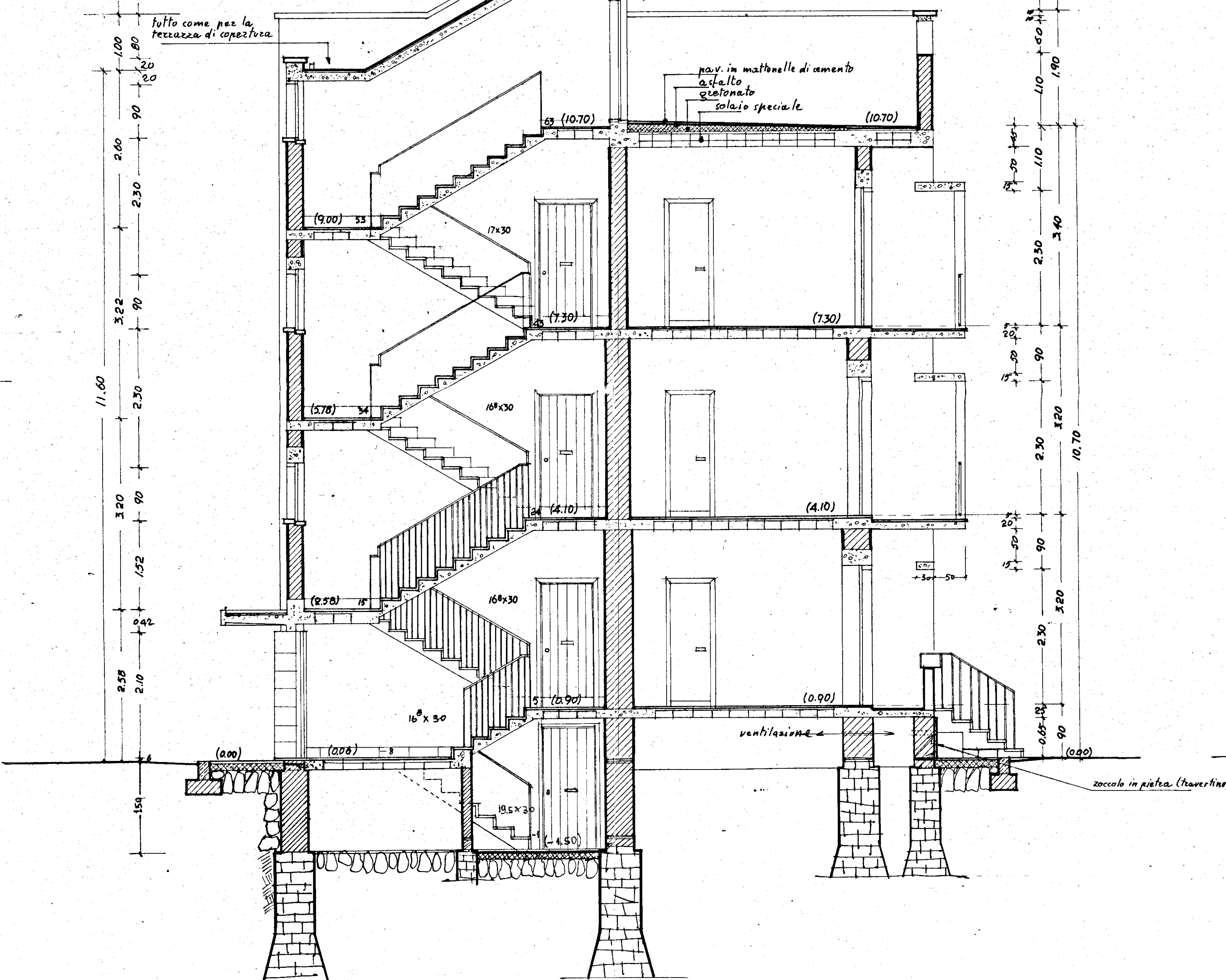
DIS. NR 183 SEZIONE D-C-B-A RAPP. 1:50
