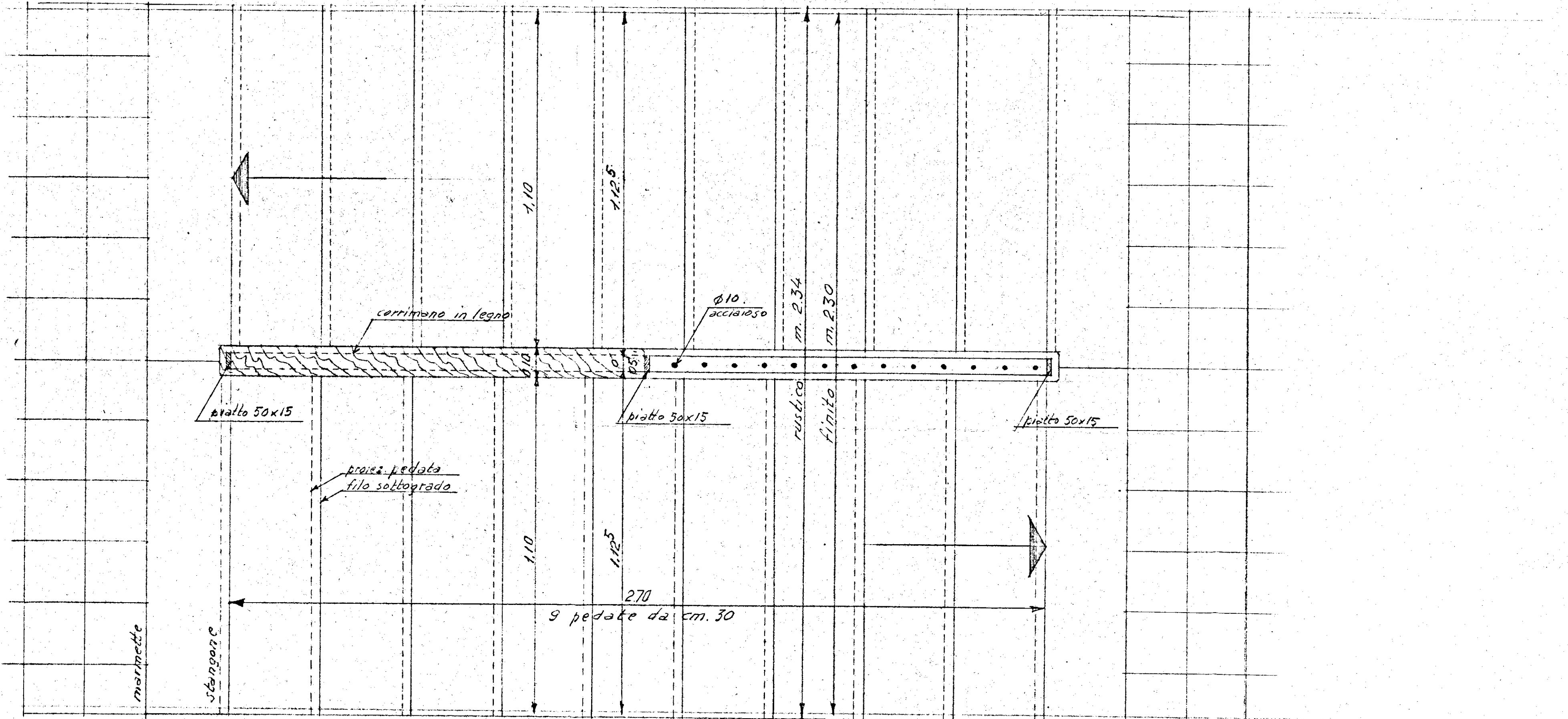
PIANTA - RAPP. 1:10
