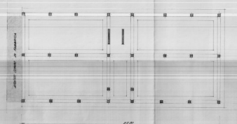
PIANTA DELLE FONDAZIONI
