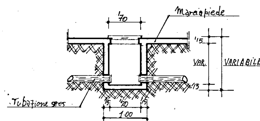
PARTICOLARE POZZETTO - 1/50
