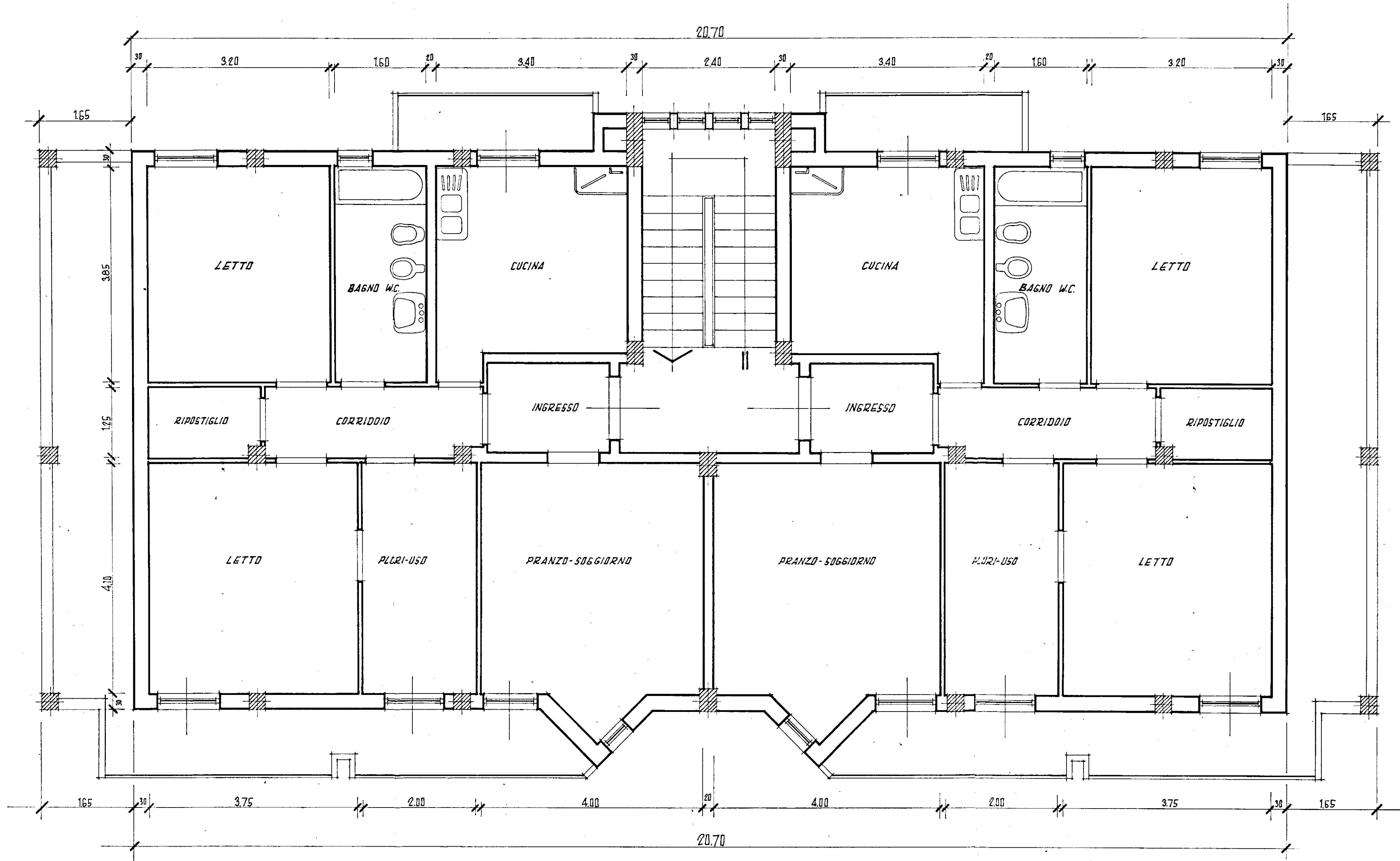
PIANTA 3° PIANO SCALA 1:50
