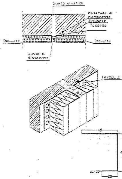
Profilo laterale utilizzato in prossimità di giunti di dilatazione
