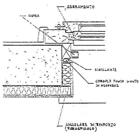
Uso del sigillante in prossimità di un vano finestra
