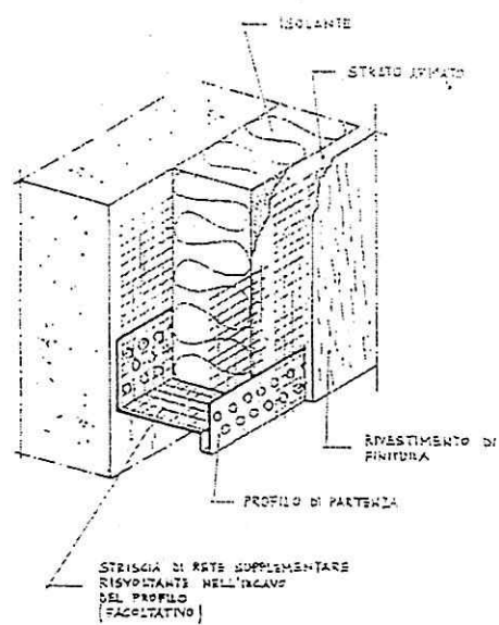
Profilo di base con gocciolatoio (o profilo di partenza)
