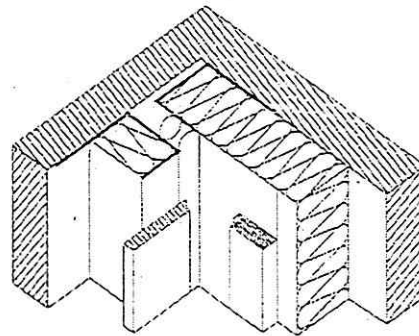
Profilo laterale utilizzato per angoli concavi
