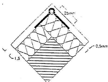
Paraspigolo (o profilo angolare di rinforzo)
