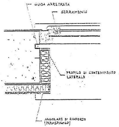
Profilo laterale utilizzato in prossimità di un vano finestra
