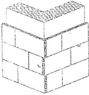
Posizionamento delle lastre agli angoli
