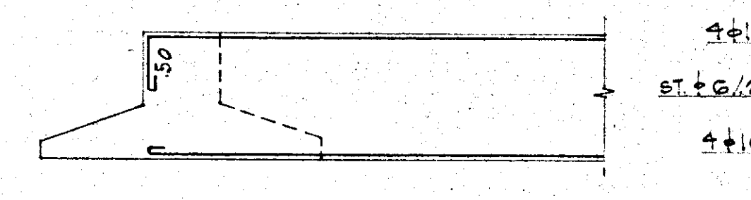
SEZIONE TIPO TRAVI DI COLLEGAMENTO
