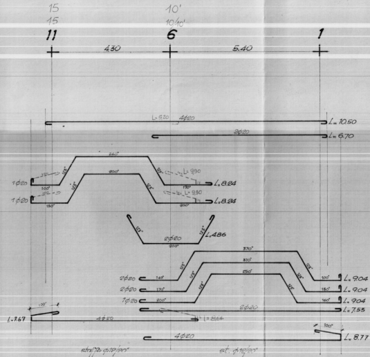
TRAVE DI TESTATA
