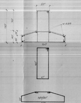
SEZIONE TRAVE TESTATA SCALA 1:20
