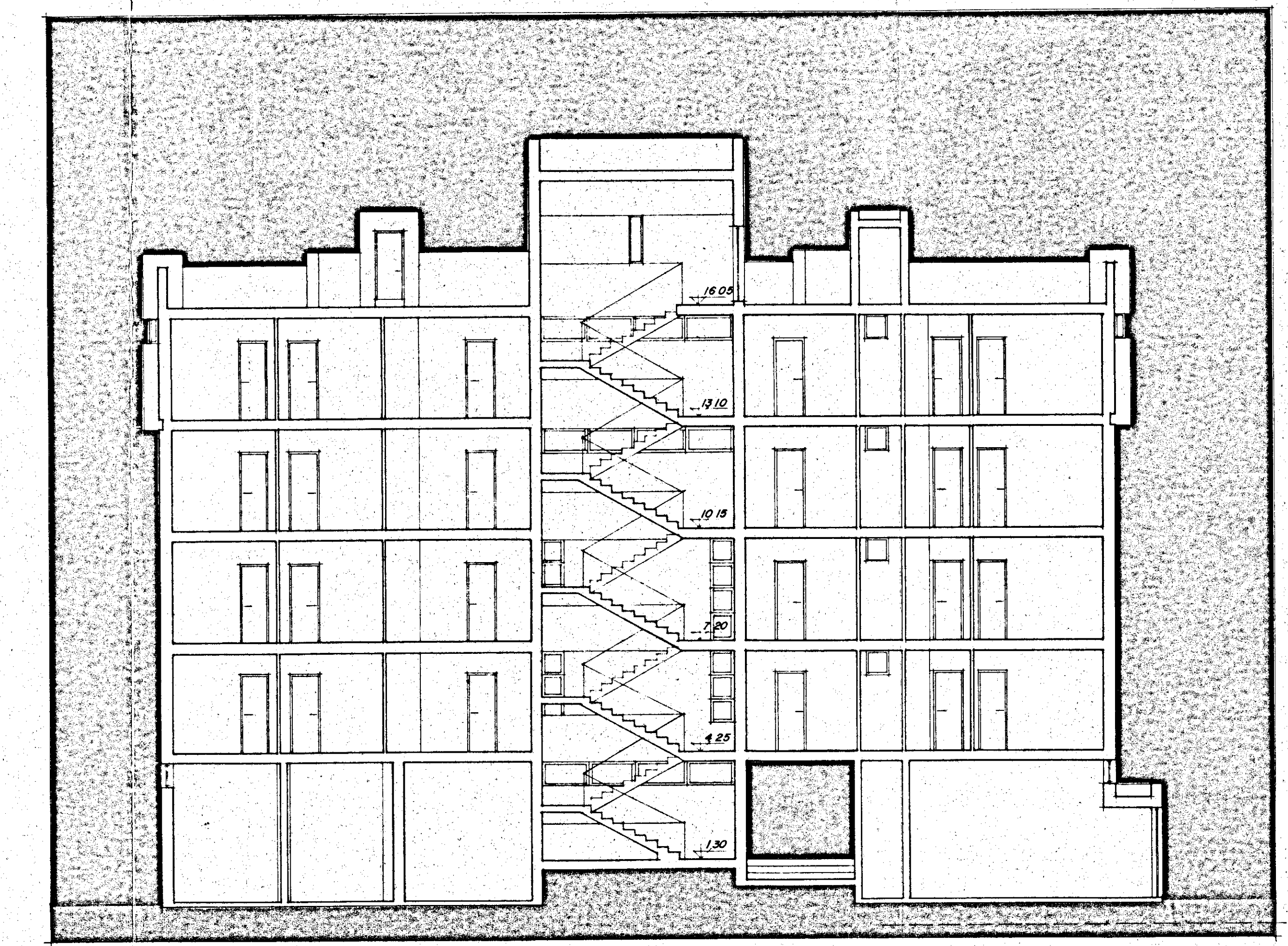
SEZIONE Y-Y
