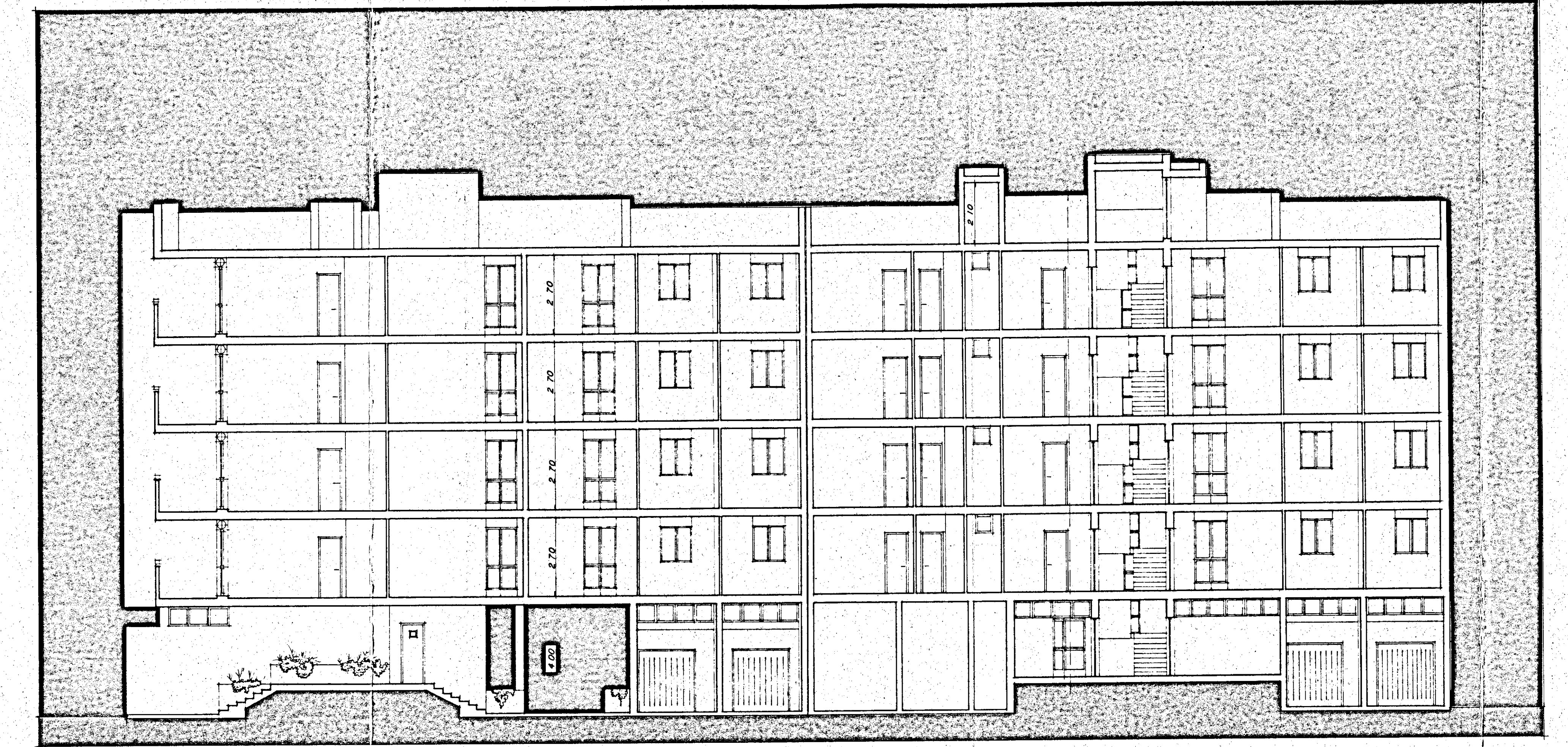
SEZIONE X-X
