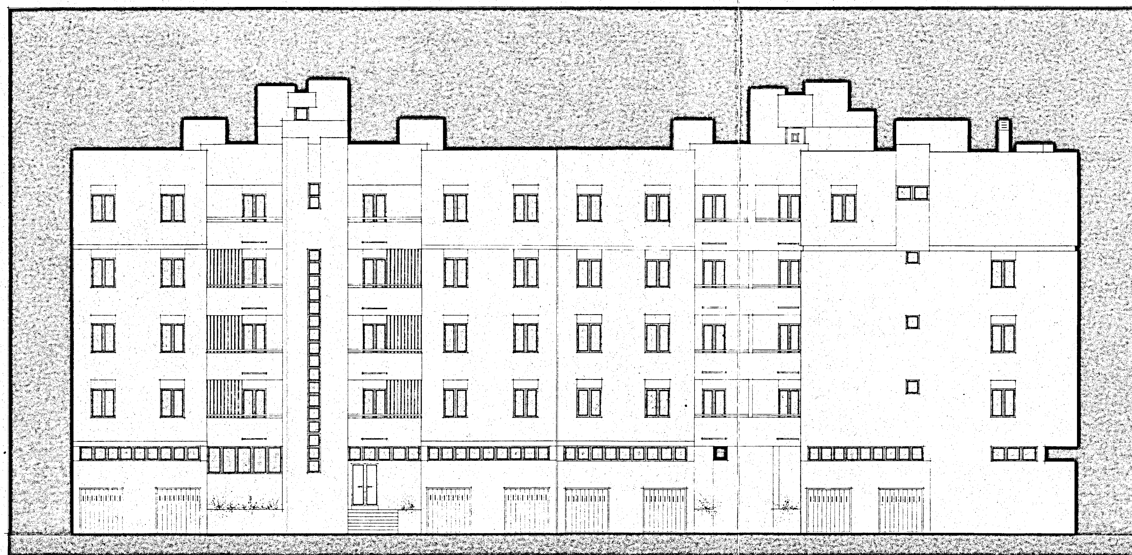
PROSPETTO -C-
