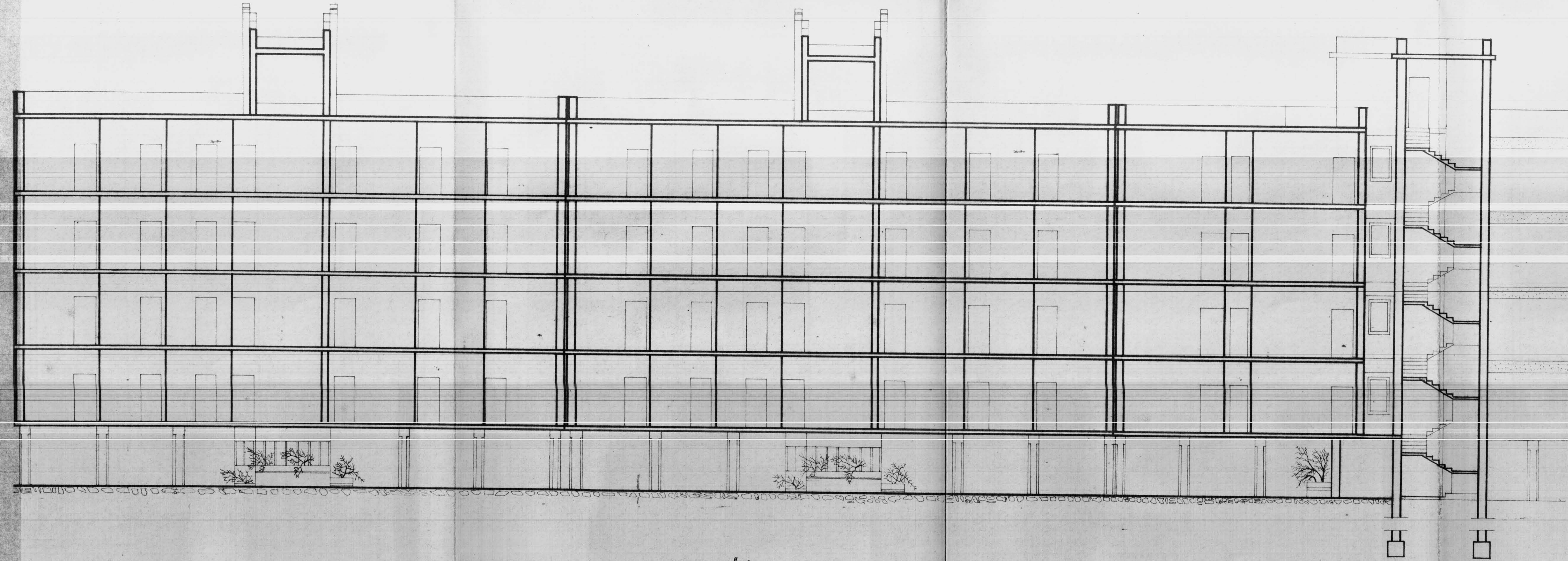
SEZIONE "AA."
