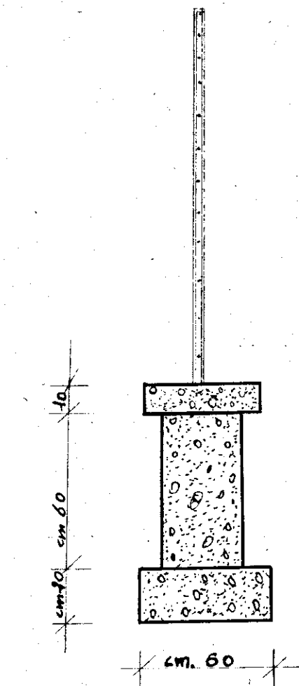
SEZ. MURO DI CINTA
