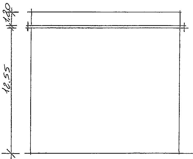
PROSPETTO M
