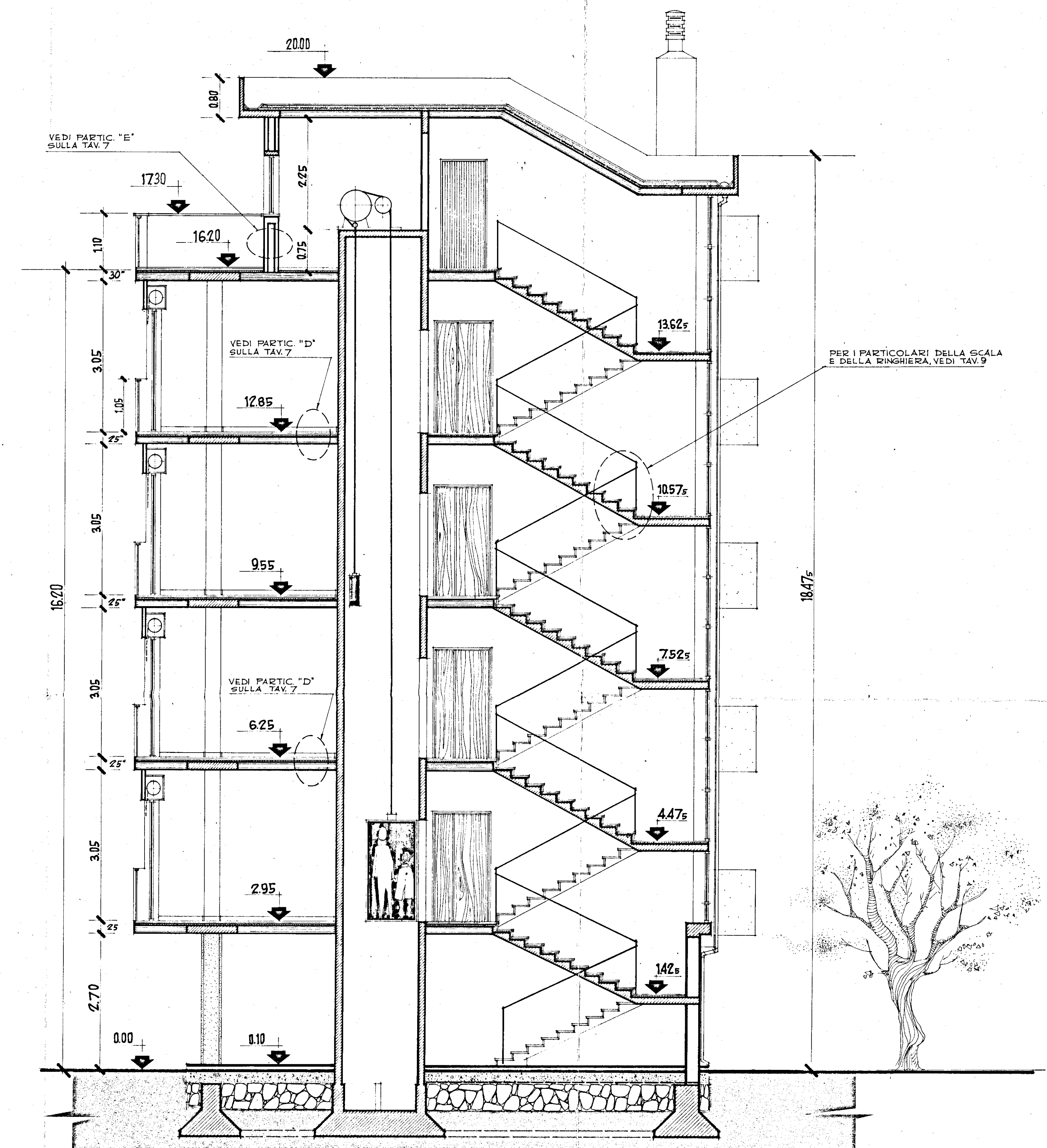
SEZIONE TRASVERSALE PALAZZINE TIPO "C" SCALA 1:50
