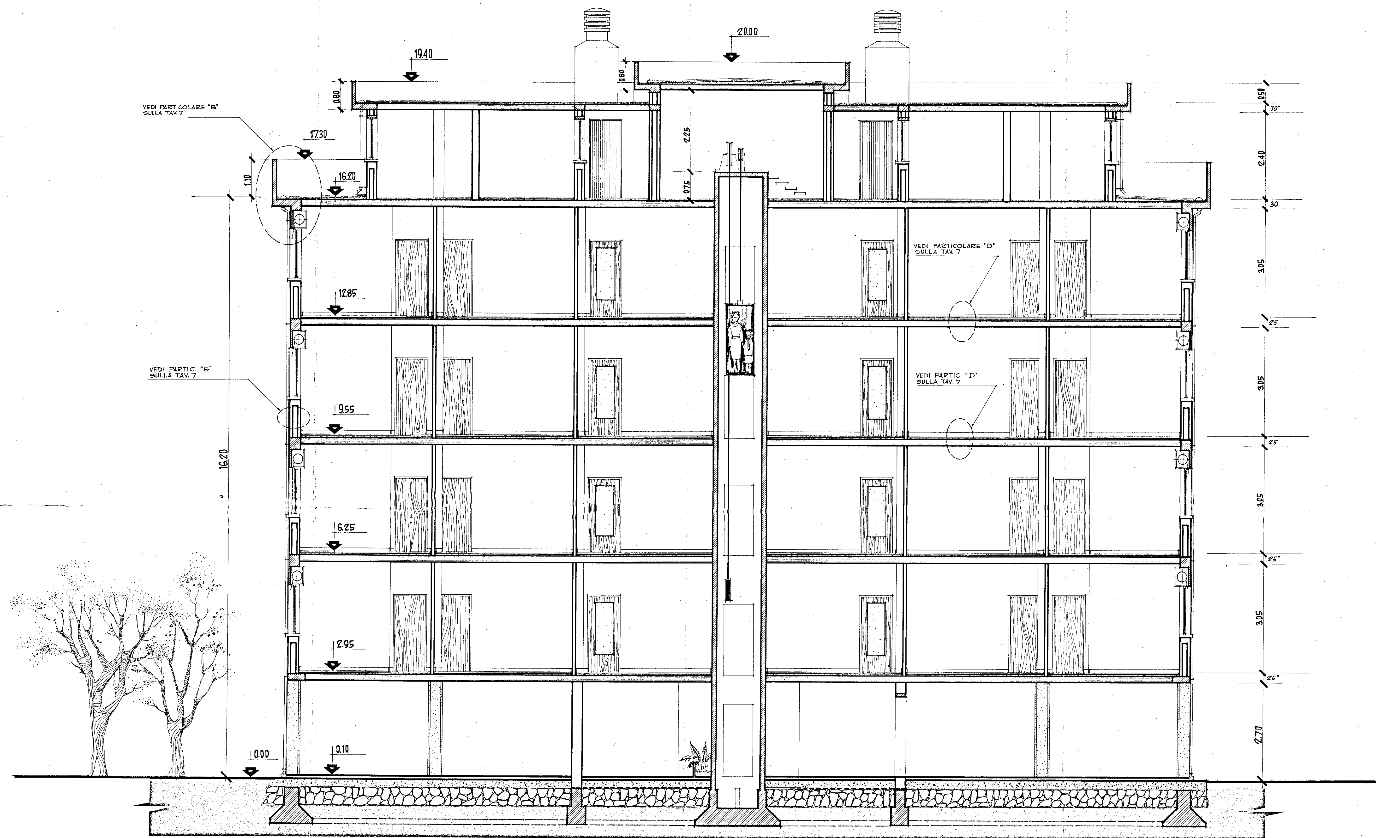
SEZIONE LONGITUDINALE PALAZZINA "D" SCALA 1:50
