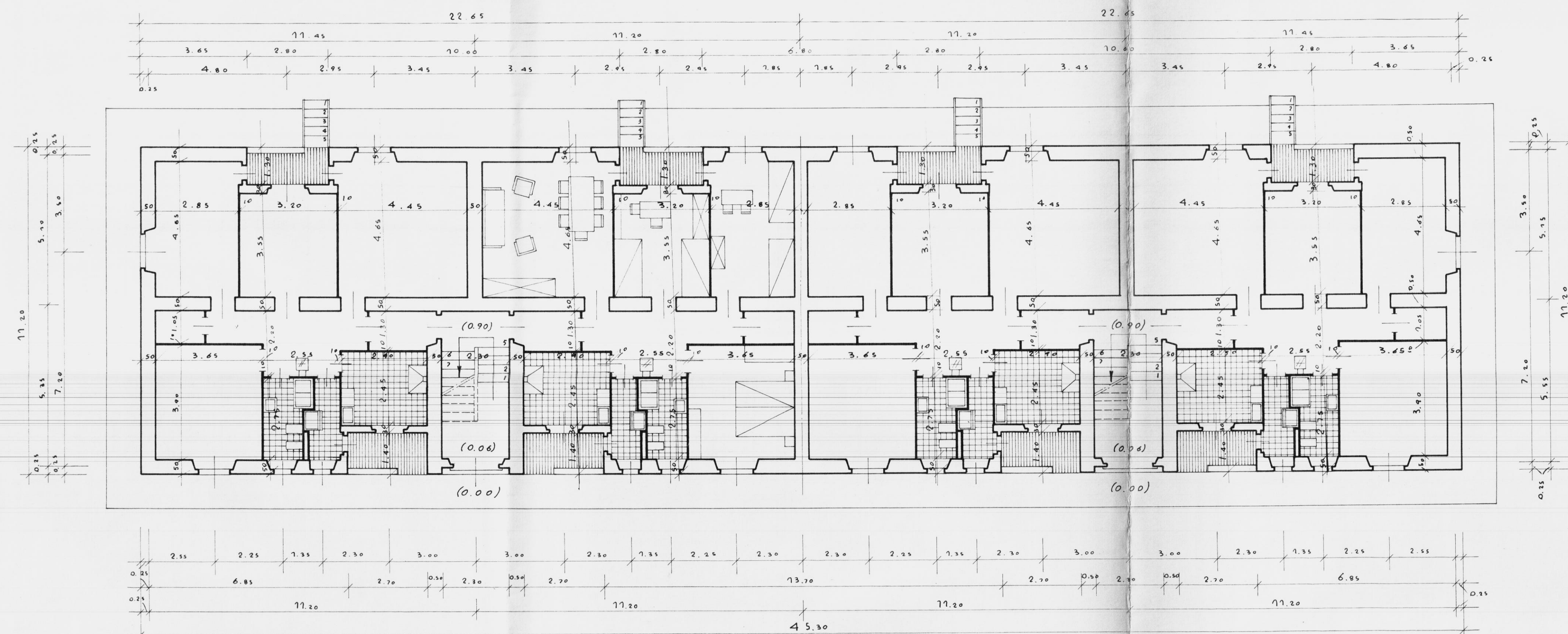
DIS. 43 PIANTE PIANO RIALZATO RAPP. 1:100
