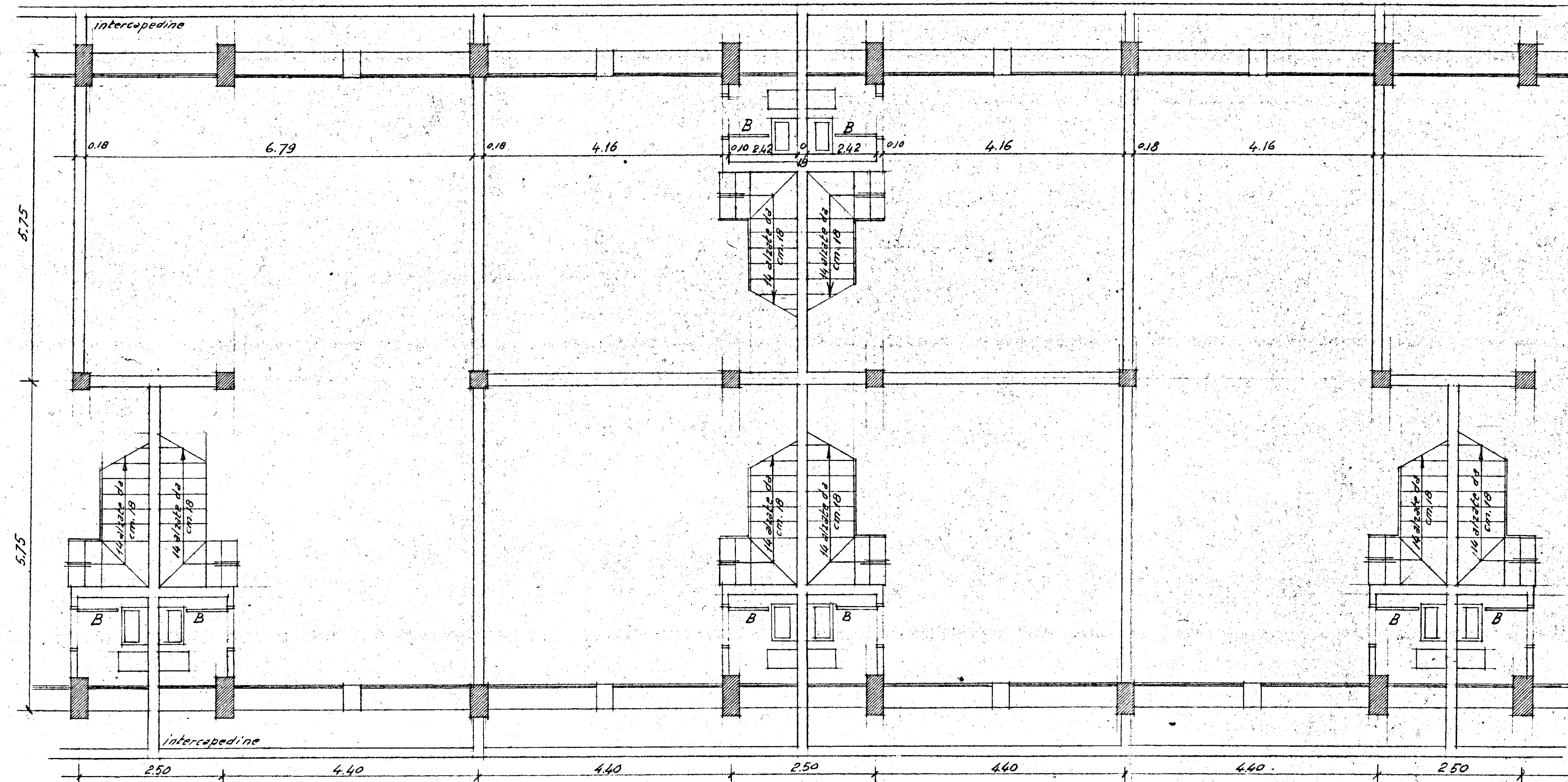
PIANTA DEL PIANO SCANTINATO NORMALE
