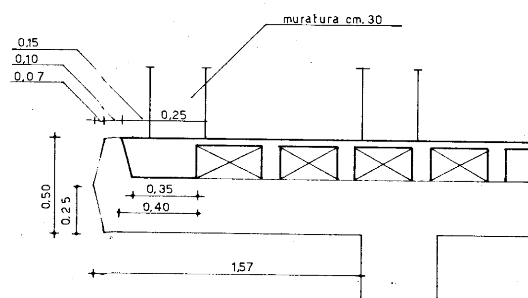
Sezione A-A rapp. 1:20
