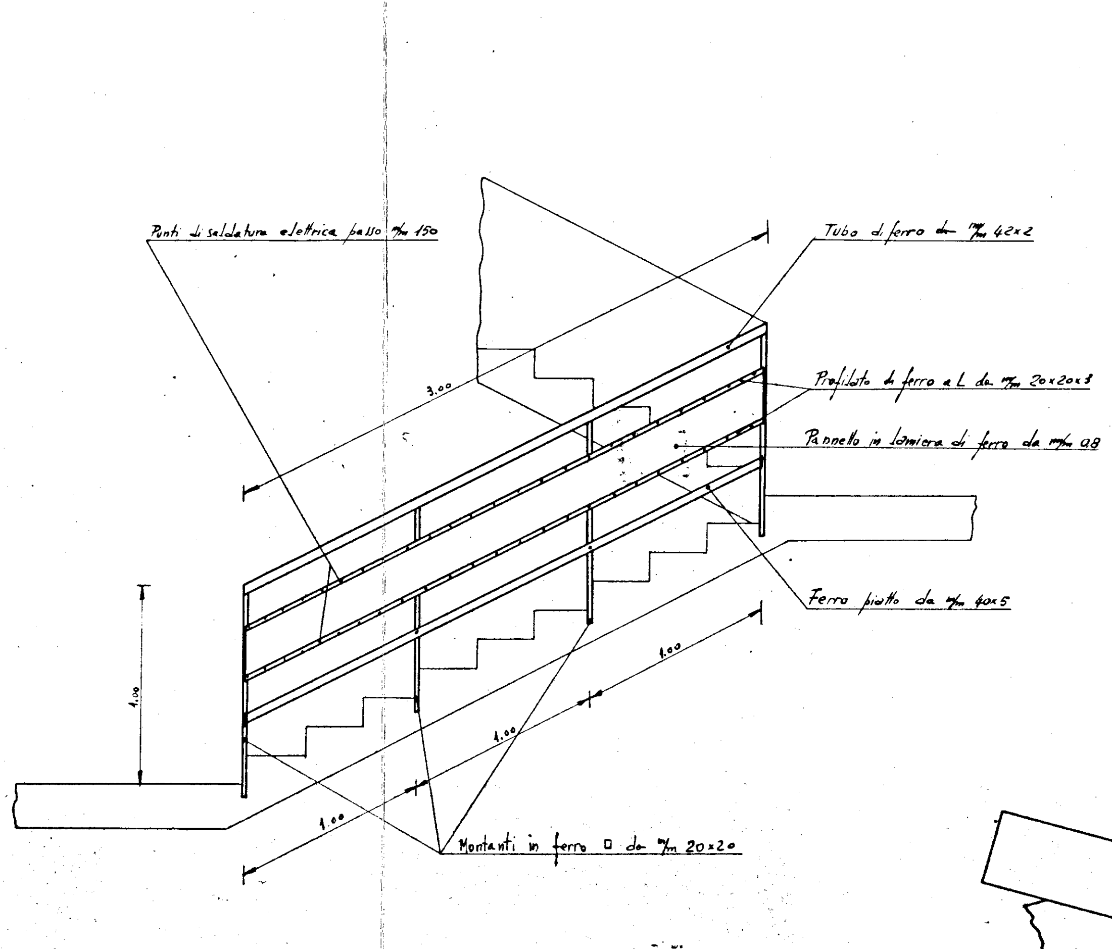
RINGHIERA PER SCALE SCALA 1:20
