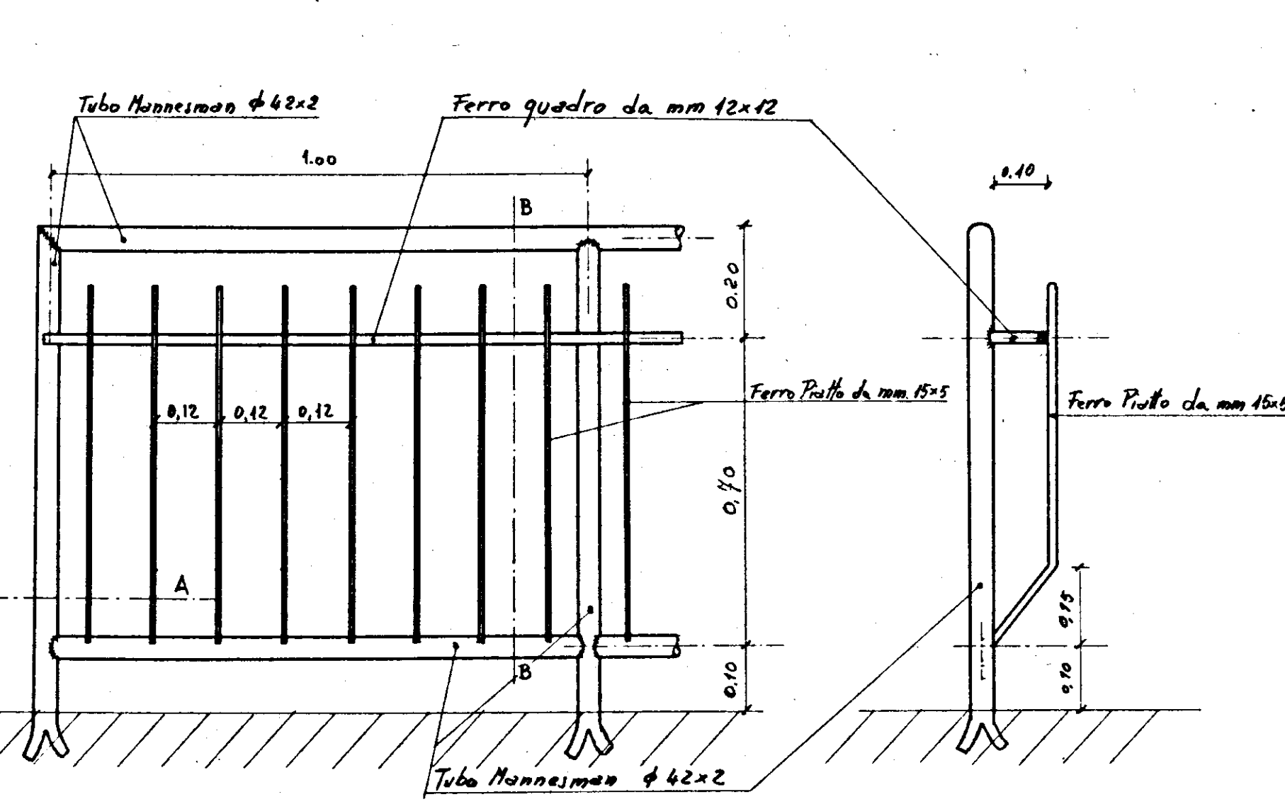
RINGHIERA PER BALCONI E VERANDE SCALA 1:10
