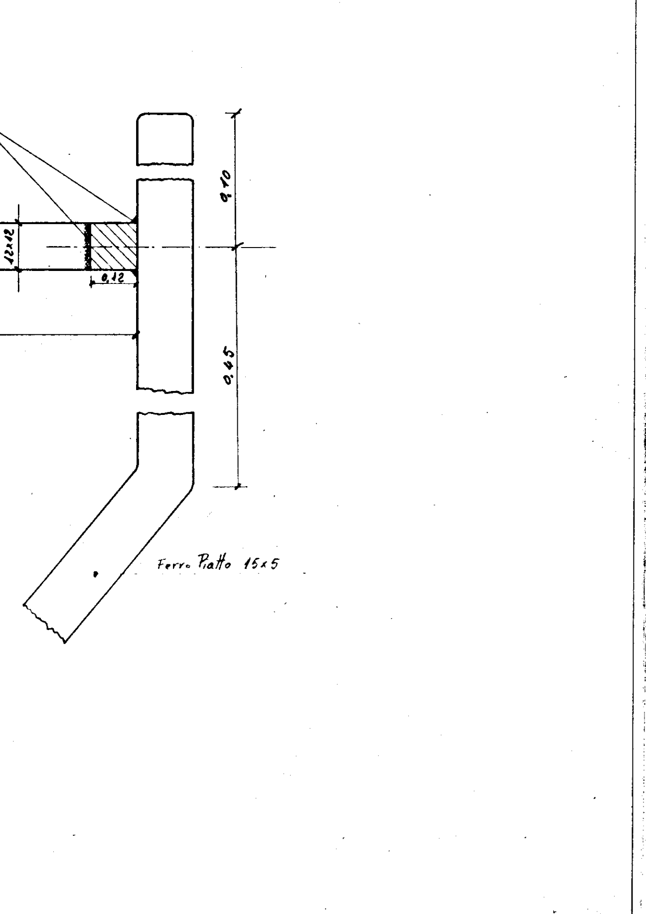
SEZ. BB SCALA 1:1
