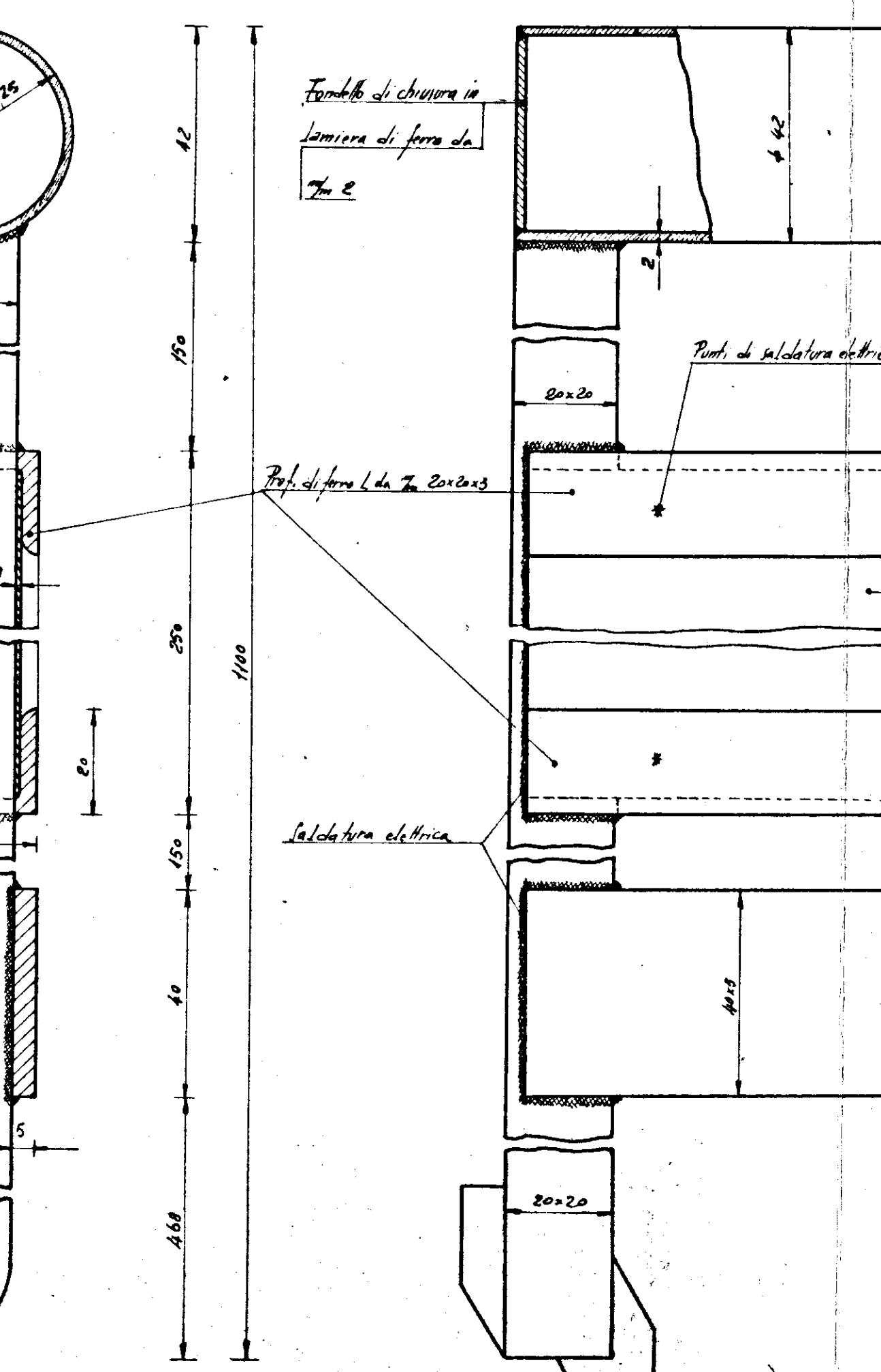
PARTICOLARE MONTANTE - SCALA 1:1
