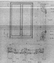
FINESTRA - TIPO CON SCURETTI -
