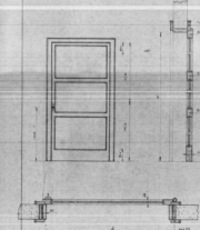
PORTA INTERNO APPARTAMENTO
