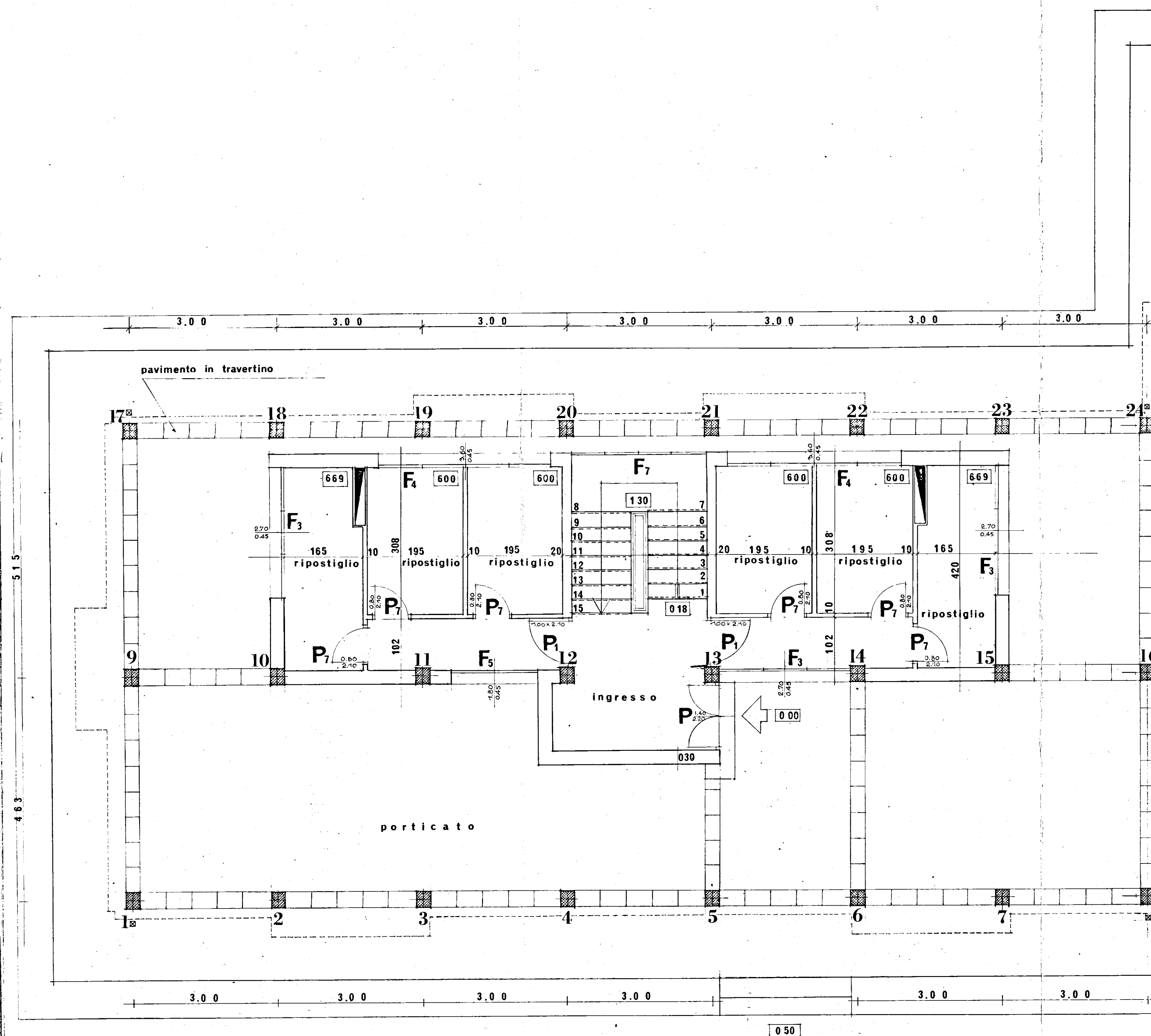
PIANTA DEL PIANO TERRENO rapp. 1:50
