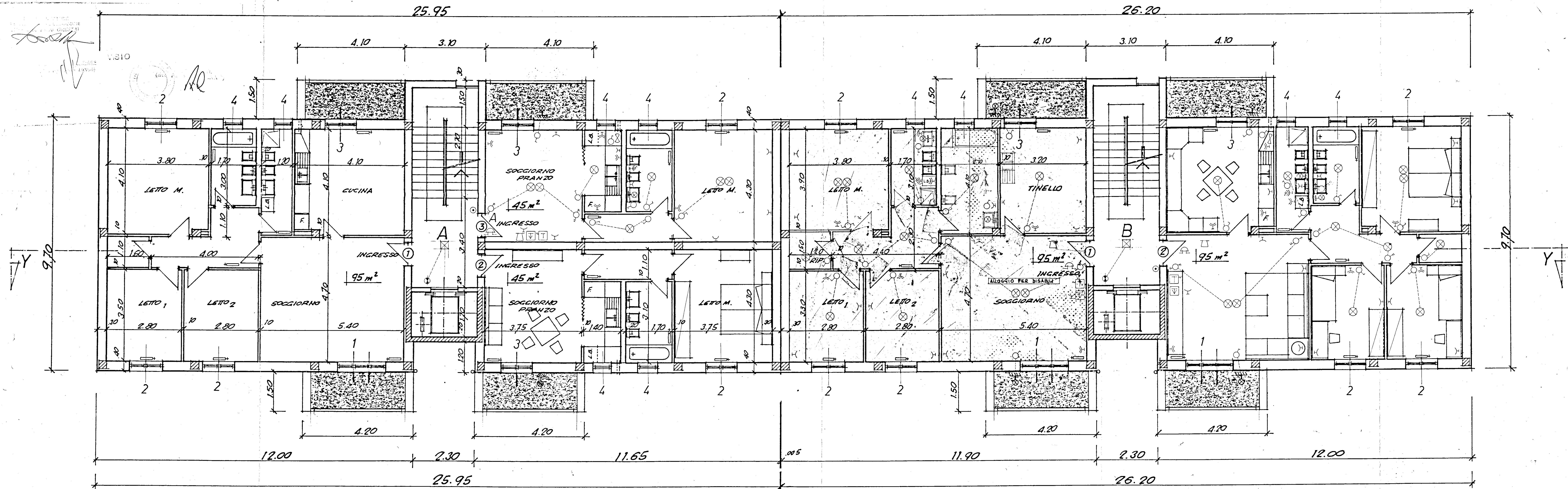
PIANTA PIANO PRIMO
