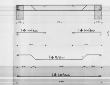
ARMATURA PIANEROTTOLO
