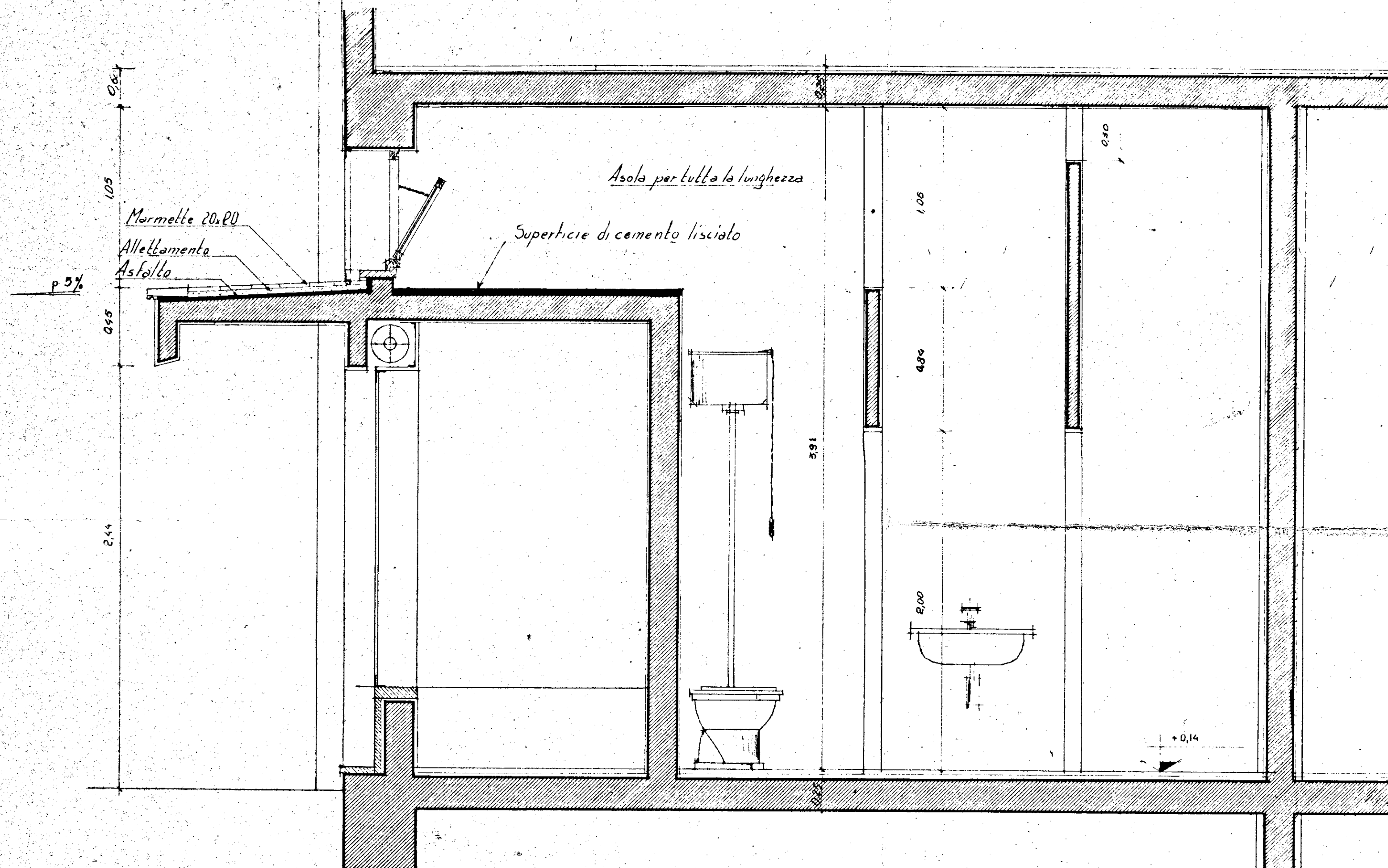
SEZIONE AA
