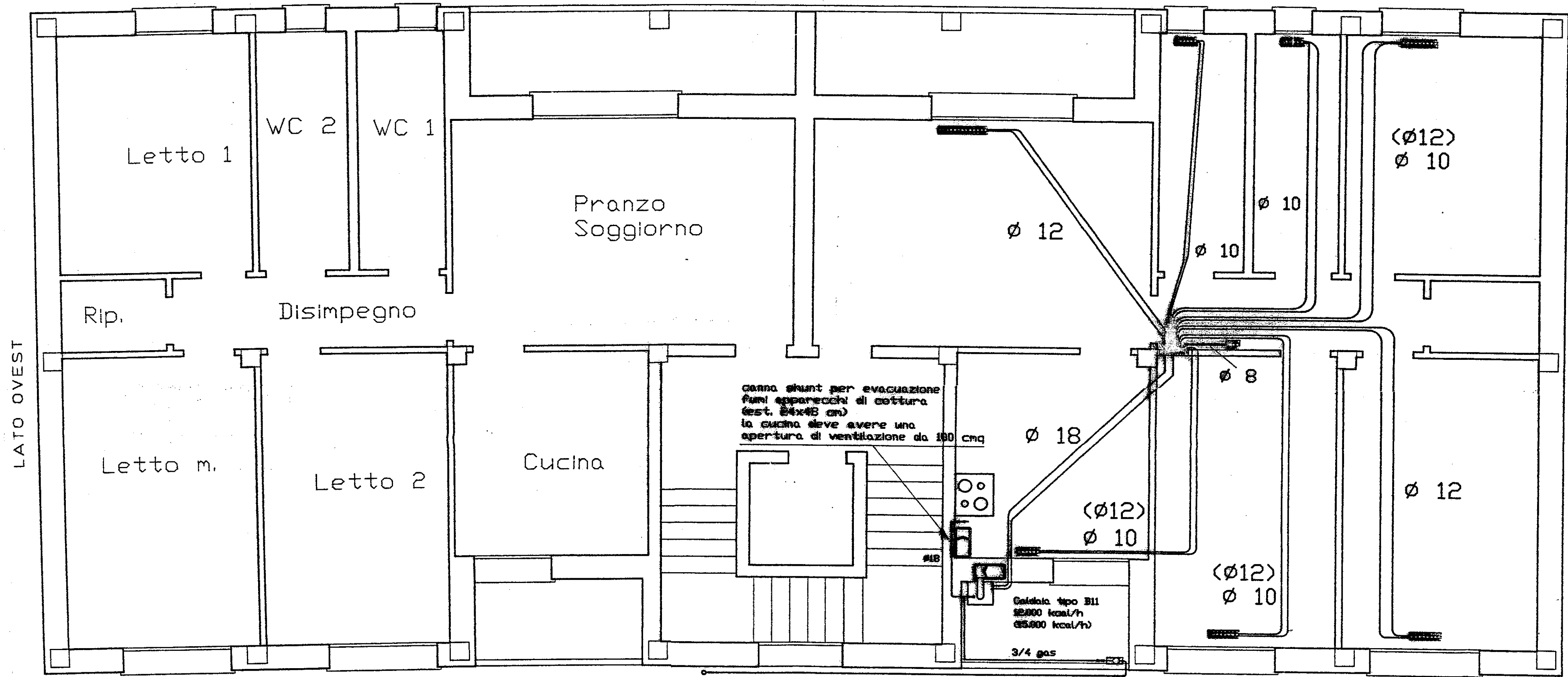
PIANO TIPO SCALA 1 : 50
